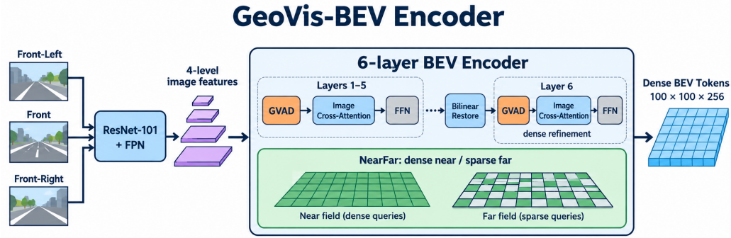
图 3: (a) GeoVis-BEV 编码器整体架构。三路前视图像经 ResNet-FPN 提取多尺度特征后输入六层编码器；GVAD 在各编码层中更新 BEV token，NearFar 在前五层保留近场稠密查询并对远场规则稀疏采样，恢复为稠密网格后由最后一层完成图像条件细化。
