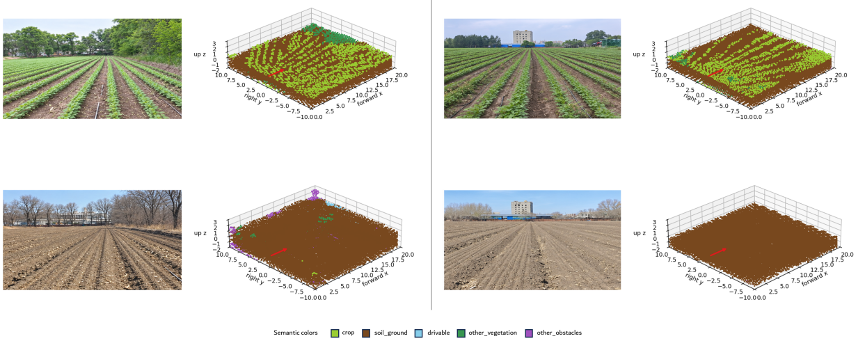
图 10: 真实农田 zero-shot 三维语义占用预测。
