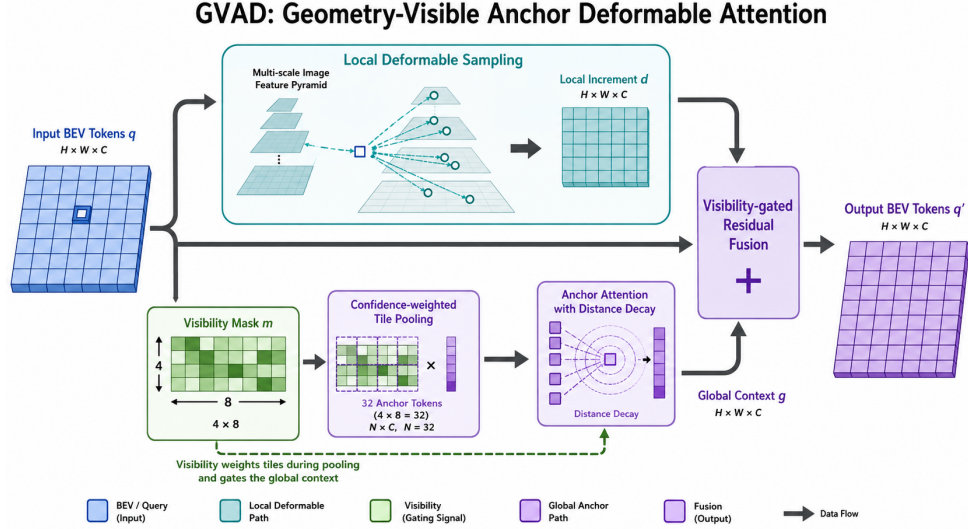
图 3: GVAD 模块。输入 BEV token 一方面在局部可变形路径中从多尺度图像读取细节, 另一方面通过可见性加权的 tile pooling 构造全局锚点; 锚点注意力与局部增量经可见性门控残差融合, 输出增强的 BEV token。
