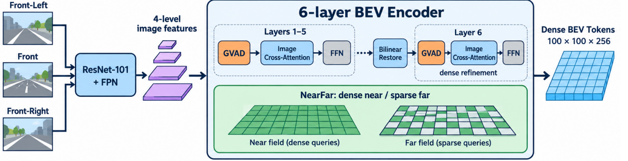
图 5: (a) GeoVis-BEV 编码器整体架构。三路前视图像经 ResNet-FPN 提取多尺度特征后输入六层编码器；GVAD 在各编码层中更新 BEV token，NearFar 在前五层保留近场稠密查询并对远场规则稀疏采样，恢复为稠密网格后由最后一层完成图像条件细化。
