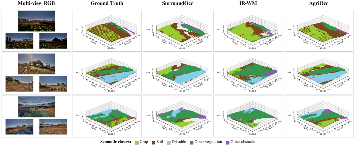
图 9: AgriOcc-Dataset 上的定性比较。每一行对应一个不同作物、光照和场景条件下的样本；从左至右依次为三路输入 RGB 图像、真值标签、SurroundOcc、IR-WM 和 AgriOcc 的当前帧三维语义占用预测。
