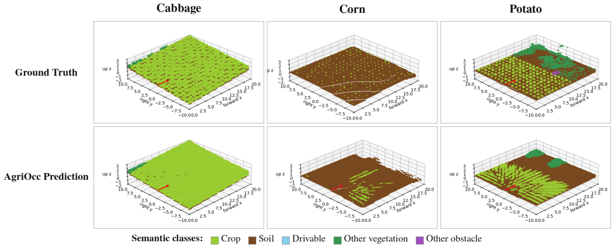
图 11: AgriOcc-Dataset 上的局限性示例。第一行为真值标签，第二行为对应的 AgriOcc 预测；三列从左至右分别为卷心菜、玉米和马铃薯场景。密集作物的株间间隙易被预测为连通区域，而苗期等小尺度作物容易出现漏检或范围不足。
