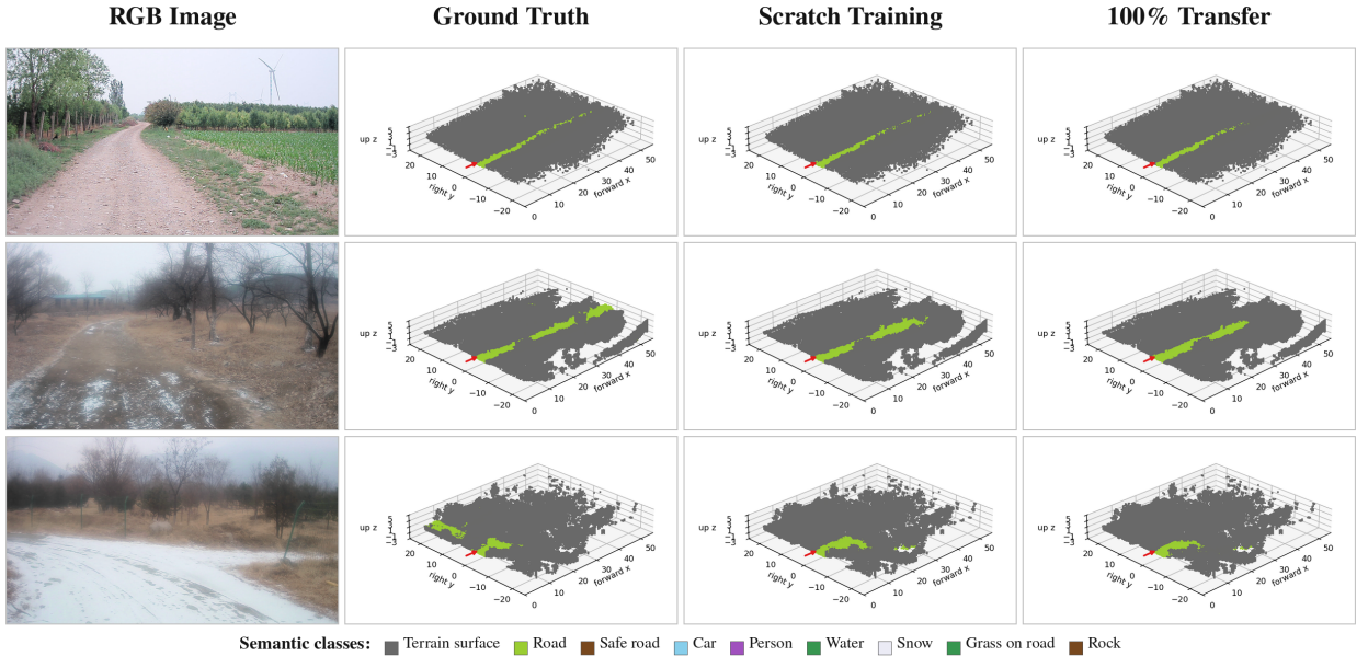
图 10: ORAD-3D 上的定性迁移比较。每行对应同一官方测试样本；从左至右为输入 RGB 图像、真值标签、使用全部 ORAD-3D 训练数据的从头训练结果，以及 AgriOcc-Dataset 预训练后在全部 ORAD-3D 训练数据上迁移的结果 (100% Transfer)。
