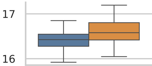
Mem avg (%)
