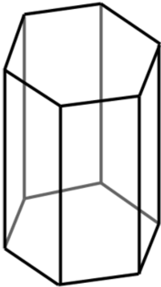
Fig: Hexagonal structure 03)6
