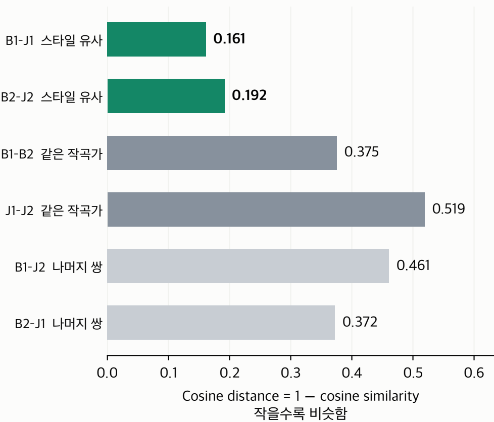
B. 원래 128차원에서의 실제 거리
