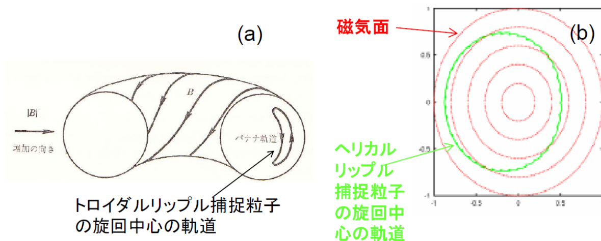
図 32 (a)トカマクにおけるトロイダルリップル捕捉粒子[7]、(b)ヘリカルにおけるヘリカルリップル捕捉粒子の軌道
