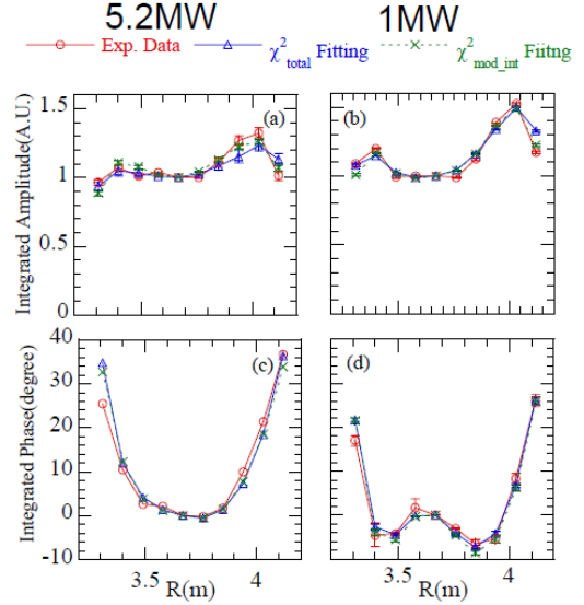
図 18 変調振幅および位相の fitting[20]
