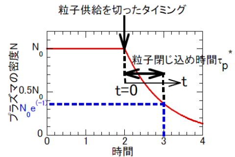
図 5 粒子閉じ込め時間の定義
