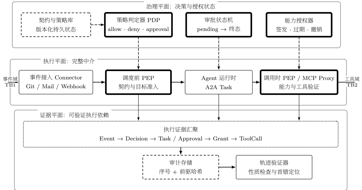
图 1: E2AG 总体架构。治理平面维护决策与授权状态，执行平面的两个 PEP 实施完整中介，证据平面记录并验证跨层对象依赖。双线框表示 E2AG 强制组件；虚线框、虚线箭头和点线箭头分别表示持久状态、治理控制和证据写入。
