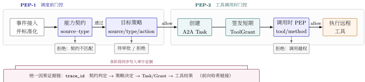
图 1: E2AG 的双执行点治理流程
