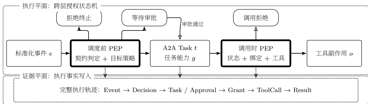
图 2: E2AG 跨层授权执行流程。两个等宽平面共享左右边界；实心箭头表示主执行路径，空心三角箭头表示治理分支，点线空心燕尾箭头表示证据写入，圆角胶囊表示暂停或终止状态。
