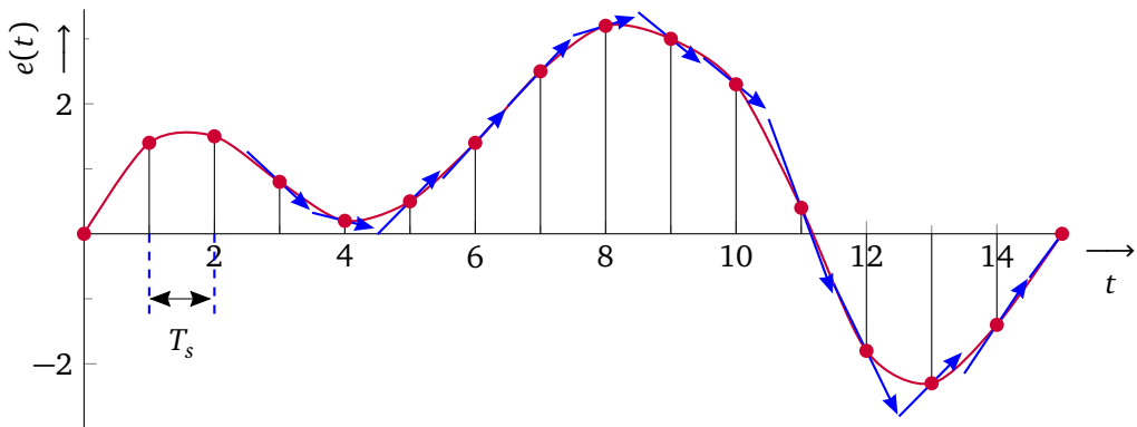
Figuur 2.7: Numeriek Differentiëren m.b.v. de vierpuntsbenadering.
