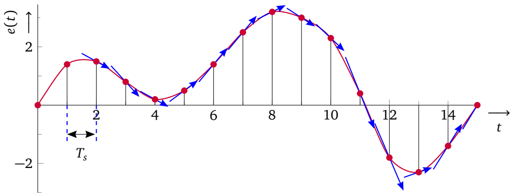
Figuur 2.6: Numeriek Differentiëren m.b.v. de driepuntsbenadering.
