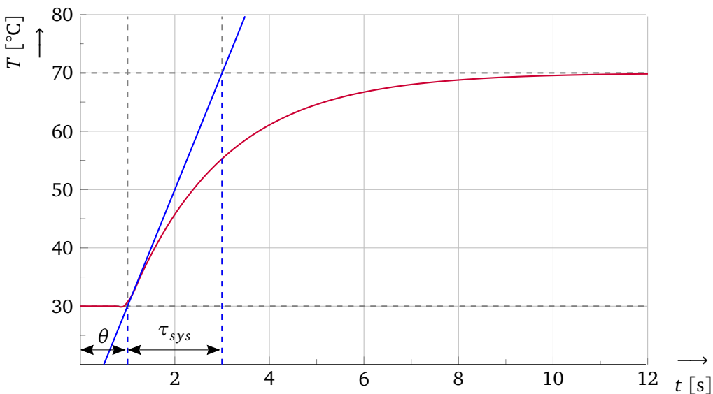
Figuur 4.1: De stapresponsie van een FOPTD.
