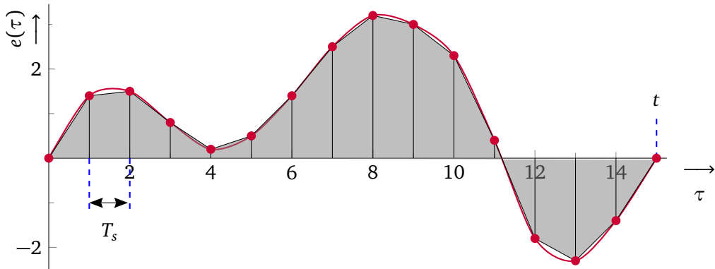
Figuur 2.4: Trapeziummethode (TRAP).
