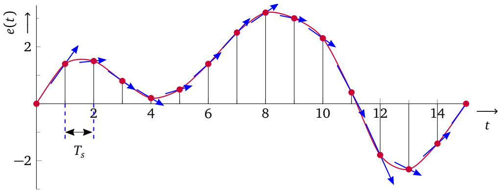
Figuur 2.5: Numeriek Differentiëren m.b.v. de tweepuntsbenadering.
