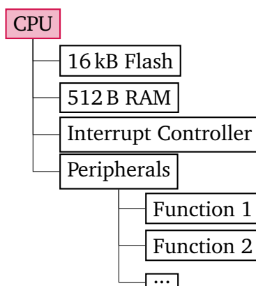
Figuur 2.1: Architectuur van een MSP430G2xxx microcontroller.
