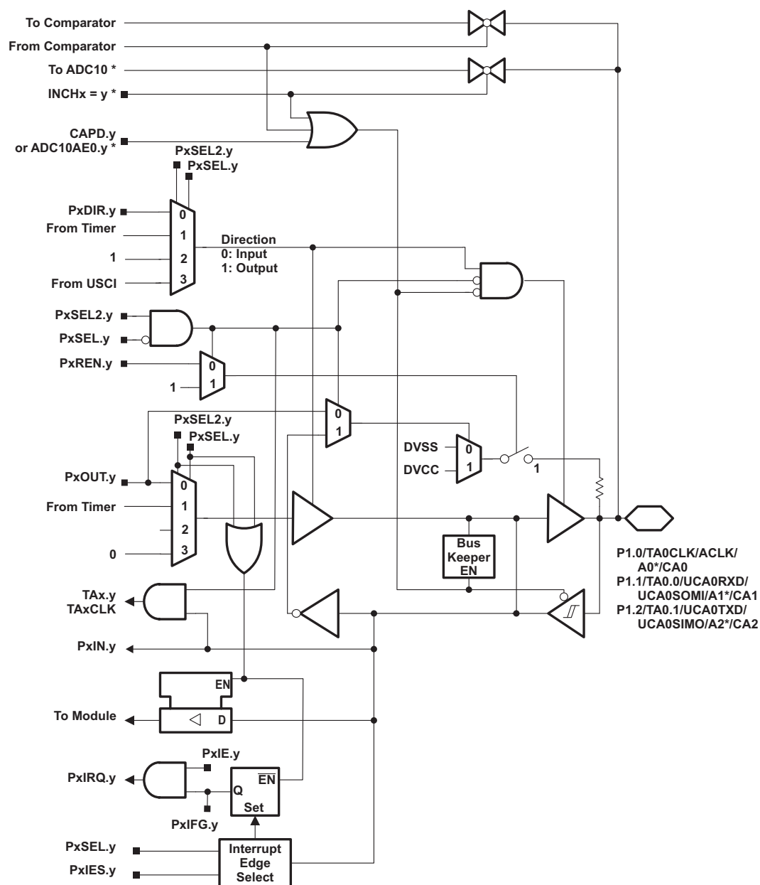
Figuur 3.1: De schakeling behorende bij P1.0 – P1.2.
