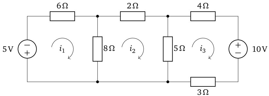
Schakeling 1: Een weerstandsnetwerk met meerdere spanningsbronnen.
