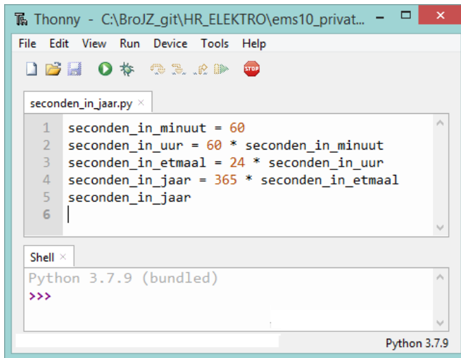
Figuur 6: Een Python script (programma) om het aantal seconden in een jaar te berekenen: seconden_in_jaar.py .
