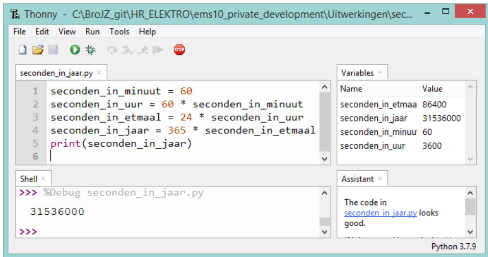
Figuur 7: In het Variables window kun je de waarden van de verschillende variabelen in je programma zien tijdens het stap voor stap uitvoeren van je programma.
