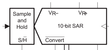
Figuur 1: Het ADC gedeelte in de \mu\text{C} (uit figuur 22-1 van de User's Guide).
