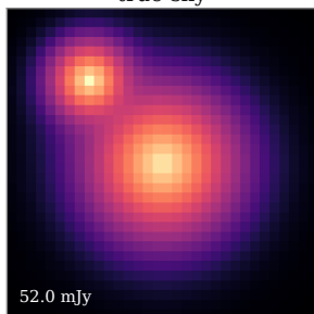
true sky
