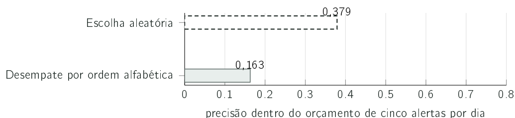
Figura 5.11: Duas formas de escolher as cinco notícias do dia, sobre o mesmo bloco de teste. O desempate alfabético não mede escolha às cegas; a escolha aleatória obtém 0,379 \pm 0,017 sobre quarenta sementes. As duas políticas escolhem conhecendo o dia completo, pelo que os valores são limites superiores do que uma política em linha consegue obter.
