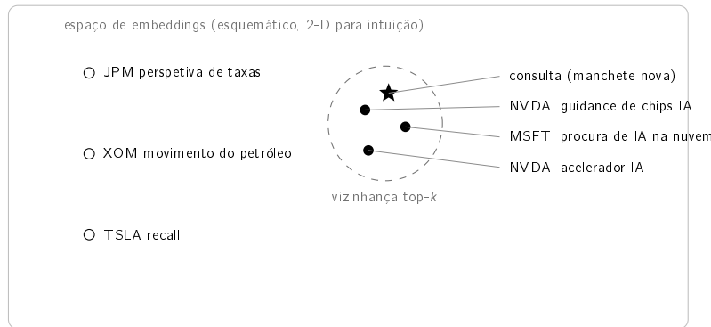
Figura 3.6: Ilustração conceitual da recuperação semântica. Cada manchete torna-se um ponto num espaço de embeddings de dimensão elevada (desenhado em duas dimensões apenas para intuição). Textos do mesmo tema ficam próximos, pelo que uma consulta (estrela) cai perto dos seus precedentes semanticamente similares (cheios), que formam a vizinhança top- k , e longe de notícias não relacionadas (ocas). A tabela seguinte torna isto concreto com números reais.
