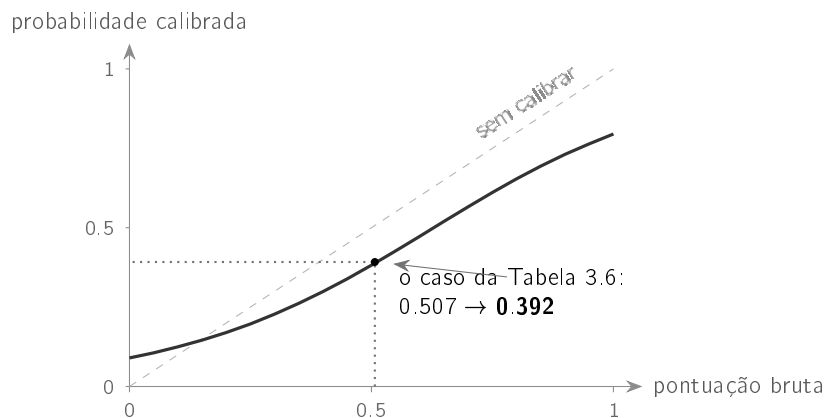
Figura 3.12: A curva que converte a pontuação do modelo numa probabilidade, com os dois valores aprendidos neste trabalho, a = 3.700 e b = -2.313 . A curva corre abaixo da diagonal em quase toda a extensão, e é isso que quer dizer o sinal negativo de b : o modelo, deixado por sua conta, anunciava mais do que acontecia, e a calibração puxa-o para baixo. O ponto marcado é o caso real seguido na Tabela 3.6, onde uma pontuação de 0.507, praticamente um lançamento de moeda, se torna 0.392.
