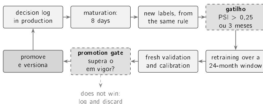
Figura 4.12: Ciclo de treino contínuo definido para este sistema e não executado no âmbito deste trabalho. O gatilho é condicional e não temporal; a janela é deslizante e a divisão permanece cronológica com embargo; e a porta de promoção impede que um modelo novo substitua o modelo em vigor sem o superar sobre um bloco reservado. A ligação a tracejado é o caminho de rejeição, e a sua existência é o que distingue o ciclo de uma automatização que persegue ruído.
