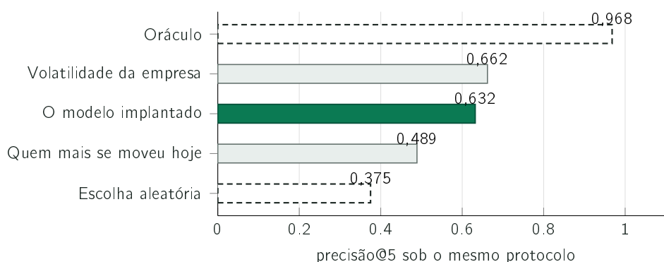
Figura 5.18: Cinco políticas de seleção sobre o mesmo bloco de teste. A escolha aleatória serve de referência; o oráculo é um máximo teórico não utilizável, obtido com conhecimento das respostas. Todas escolhem conhecendo o dia completo, pelo que cada valor é um limite superior do que a mesma regra obteria decidindo ao minuto.
