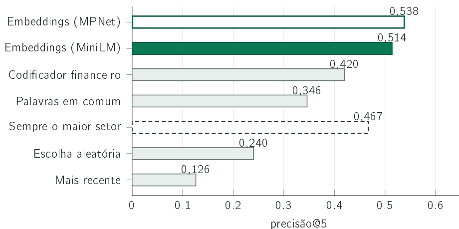
Figura 5.6: Precisão@5 do MiniLM implantado, em verde cheio, contra seis alternativas. O contorno verde identifica a variante MPNet de maior dimensão; as barras cinzentas reúnem duas linhas de base, uma linha lexical e um codificador específico do domínio financeiro. A alternativa tracejada de devolver sempre notícias do setor maior obtém 0,467 sem qualquer modelo, valor discutido no texto e que obriga a ler o agregado com reserva.
