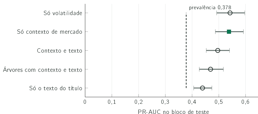
Figura 5.9: Área sob a curva de precisão e cobertura de cinco modelos, com intervalos marginais a noventa e cinco por cento obtidos por reamostragem dos 1 951 grupos. A linha tracejada assinala a prevalência do bloco de teste, que é o valor obtido por um modelo que atribua a mesma probabilidade a todos os exemplos. Os valores são pontos, e os intervalos são amplos e sobrepõem-se: [0,492; 0,597] para a volatilidade, [0,487; 0,592] para o contexto e [0,453; 0,540] para o contexto com texto. A comparação que a subsecção seguinte sustenta é a diferença emparelhada entre modelos sobre as mesmas reamostragens, e não a distância entre dois pontos.
