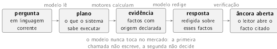
Figura 4.13: As duas chamadas ao modelo de linguagem estão separadas de propósito. A primeira traduz uma frase humana num plano que o sistema sabe executar e não escreve texto. A segunda redige sobre factos que já existem e não decide nada. Entre as duas, os motores descritos neste capítulo produzem a evidência, e cada facto chega com a origem declarada. A verificação final recusa a frase cujo número não pertença ao facto que ela cita, e é o que permite ao leitor abrir a âncora e confrontar a afirmação com aquilo que a sustenta.
