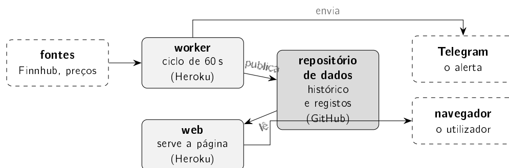
Figura 4.5: Os dois processos do Heroku não partilham disco. Tudo o que tem de sobreviver a um reinício, ou de ser visto pelo outro processo, passa pela branch de dados no GitHub.
