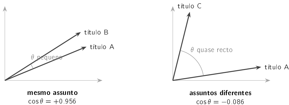
Figura 3.8: Cada título é uma seta com 384 coordenadas, aqui desenhada em duas para se poder ver. O que se compara é o ângulo entre elas, e não o sítio onde as pontas caem: um título curto e um parágrafo longo sobre o mesmo assunto apontam na mesma direção, e o comprimento da seta, que é o que a distância mediria, diz respeito ao tamanho do texto e não ao seu tema. Os dois valores são os do par real da Tabela 3.5.
