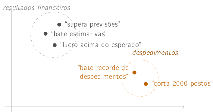
Figura 3.7: Cada frase vira um ponto. Frases com o mesmo significado ficam próximas, mesmo sem partilharem palavras; frases que partilham palavras (“bate”) mas falam de assuntos diferentes ficam longe. O desenho tem duas dimensões para se poder ver; o modelo usa 384.
