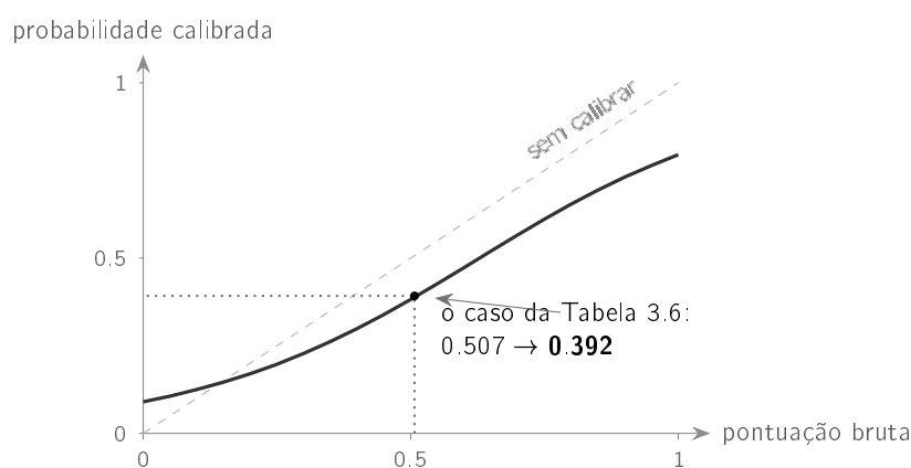
Figura 3.12: A curva que converte a pontuação do modelo numa probabilidade, com os dois valores aprendidos neste trabalho, a = 3.700 e b = -2.313 . A curva corre abaixo da diagonal em quase toda a extensão, e é isso que quer dizer o sinal negativo de b : o modelo, deixado por sua conta, anunciava mais do que acontecia, e a calibração puxa-o para baixo. O ponto marcado é o caso real seguido na Tabela 3.6, onde uma pontuação de 0.507, praticamente um lançamento de moeda, se torna 0.392.
