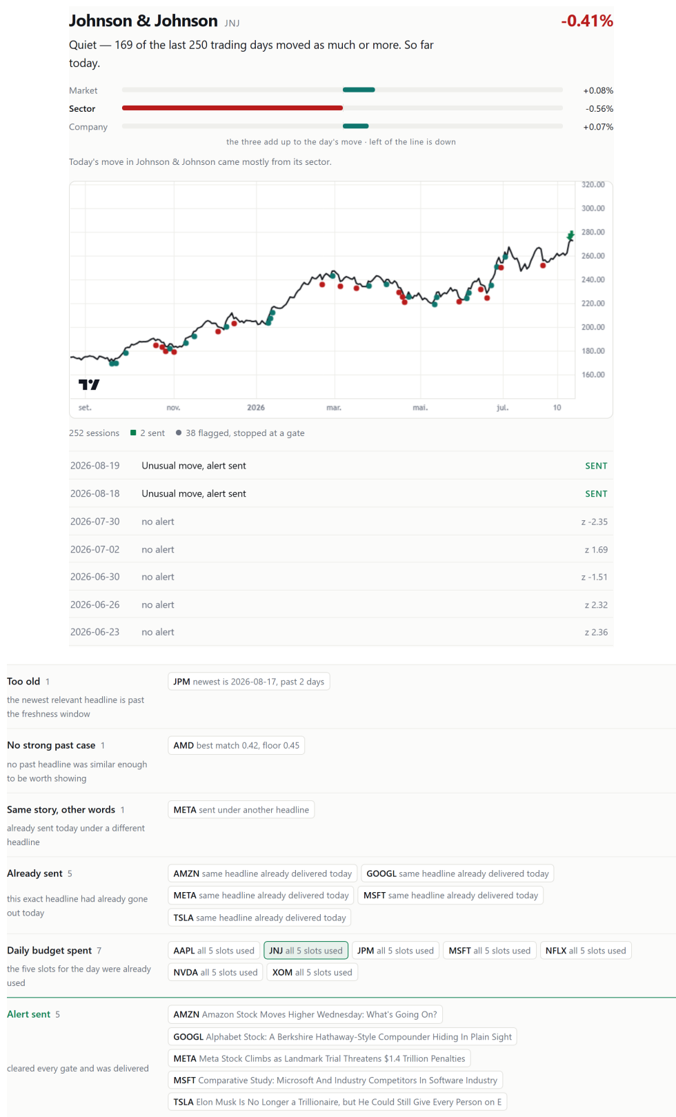
Figura 4.4: A página, capturada da aplicação em funcionamento a 20 de agosto de 2026, com a sessão americana a decorrer. Em cima , uma empresa. Em baixo , as decisões do dia inteiro, pela ordem por que são tomadas, com a margem que faltou quando existe.
