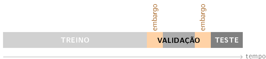
Figura 3.11: Os dados são divididos por ordem cronológica , nunca ao acaso. Entre blocos há um embargo de cinco dias, porque o rótulo de uma notícia olha até três dias para a frente e sem o embargo o fim do treino tocava no princípio do teste.
