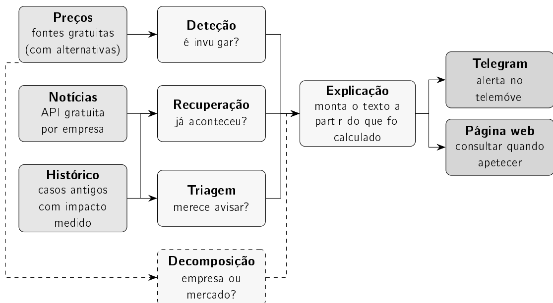
Figura 4.1: As cinco partes do InvestiGator. À esquerda, de onde vêm os dados; ao centro, as quatro técnicas do capítulo anterior mais o motor que compõe o texto; à direita, as duas formas de o utilizador receber o resultado. A decomposição está a tracejado porque é a única que não corre em todos os alertas: só entra no de preço, já que sem movimento do dia não há nada para repartir.
