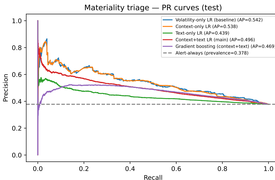
Figura 5.7: As curvas sobre o bloco de teste. A área debaixo de cada curva é o valor da tabela. A curva do modelo que usa apenas volatilidade está por cima das outras em quase toda a extensão, e não só no valor agregado.
