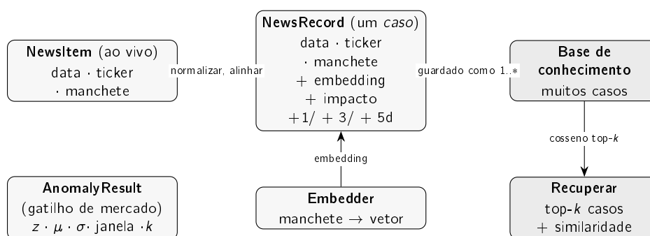
Figura 4.3: Os objetos com que o InvestiGator trabalha. Um NewsItem ao vivo e um NewsRecord histórico partilham o mesmo esquema (data, ticker, manchete); um NewsRecord é um caso , acrescentando o embedding da manchete e o seu impacto medido pós-evento. O Embedder produz esses vetores; a Base de conhecimento guarda muitos casos; uma manchete de consulta recupera os top- k casos mais similares com as suas pontuações de similaridade. O gatilho de mercado produz um AnomalyResult separado.
