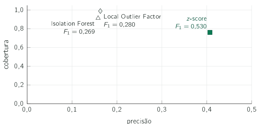
Figura 5.3: Os três detetores sobre os mesmos dados e sob o mesmo protocolo, restrito à região que os três conseguem pontuar. Os dois métodos aprendidos ocupam a região de cobertura quase total e precisão baixa; a regra troca alguma cobertura por precisão. O F_1 junto de cada ponto resume esse compromisso. A amplitude da taxa de disparo acompanha o mesmo padrão, com 0,017 para a regra contra 0,140 e 0,183 para os detetores aprendidos.
