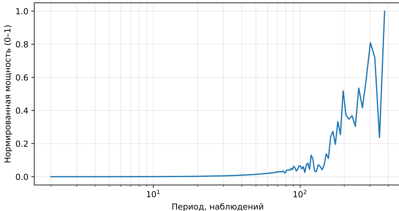
Нормированный спектр реконструкции (AE), price, тикер: SNPS
