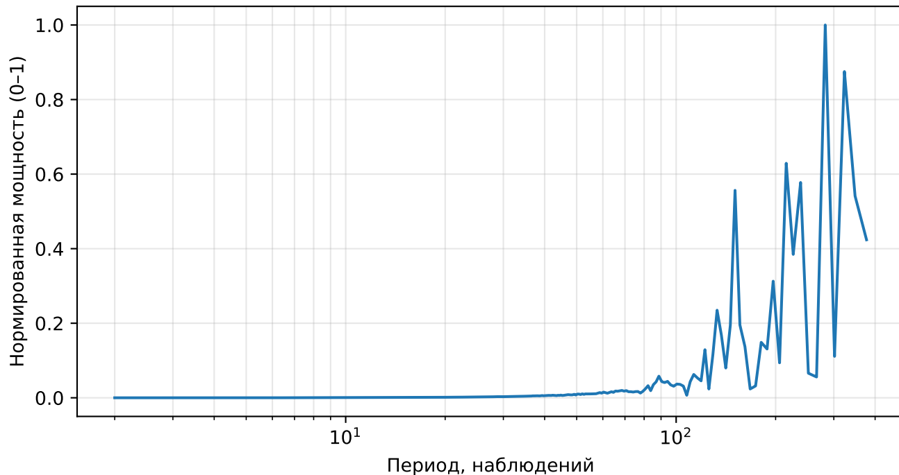
Нормированный спектр реконструкции (AE), price, тикер: CVS
