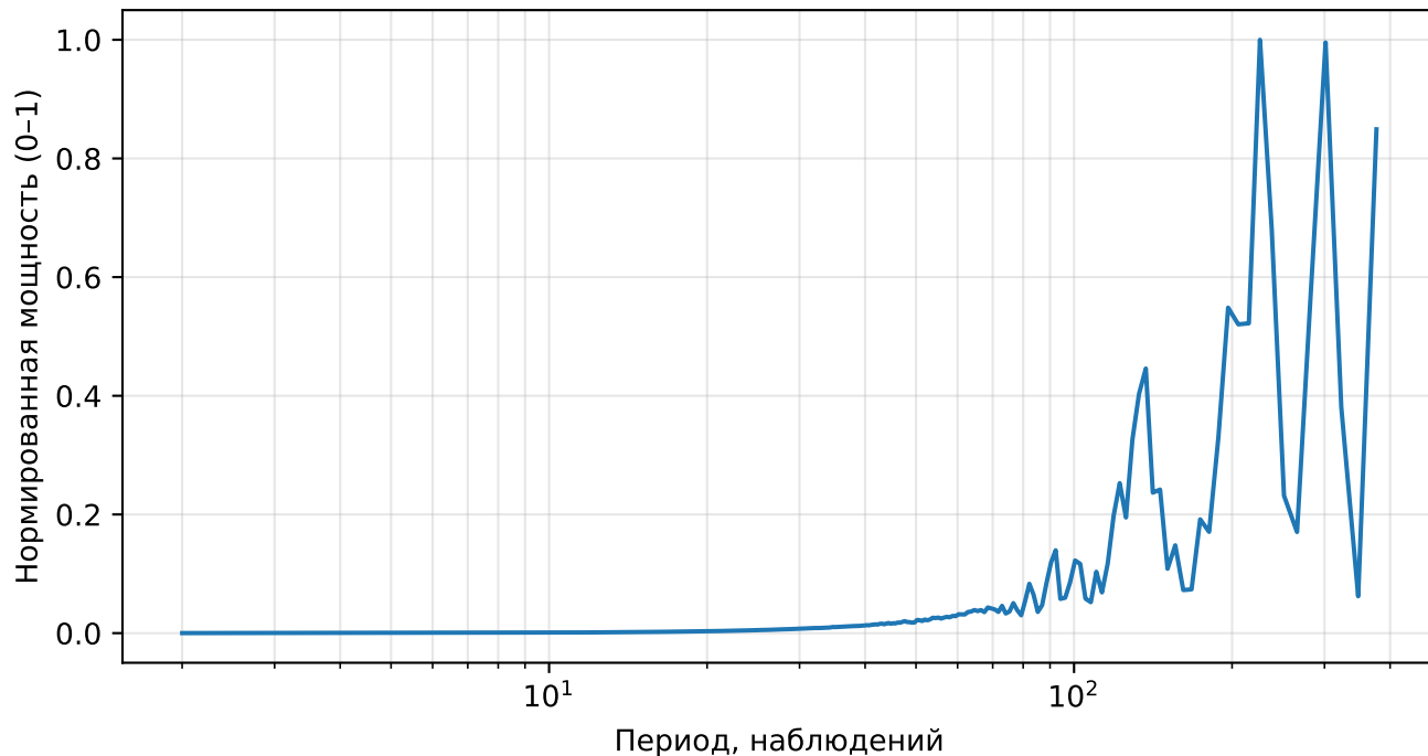
Нормированный спектр реконструкции (AE), price, тикер: ICE
