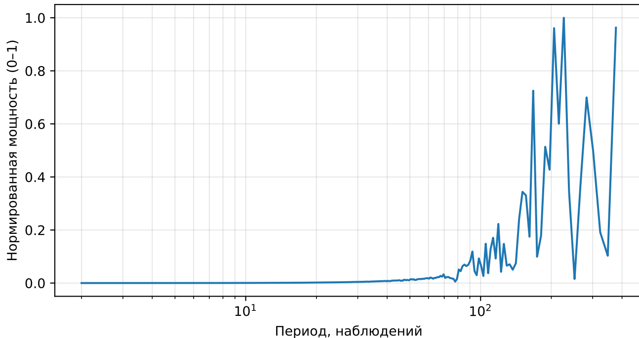
Нормированный спектр реконструкции (AE), price, тикер: INTC
