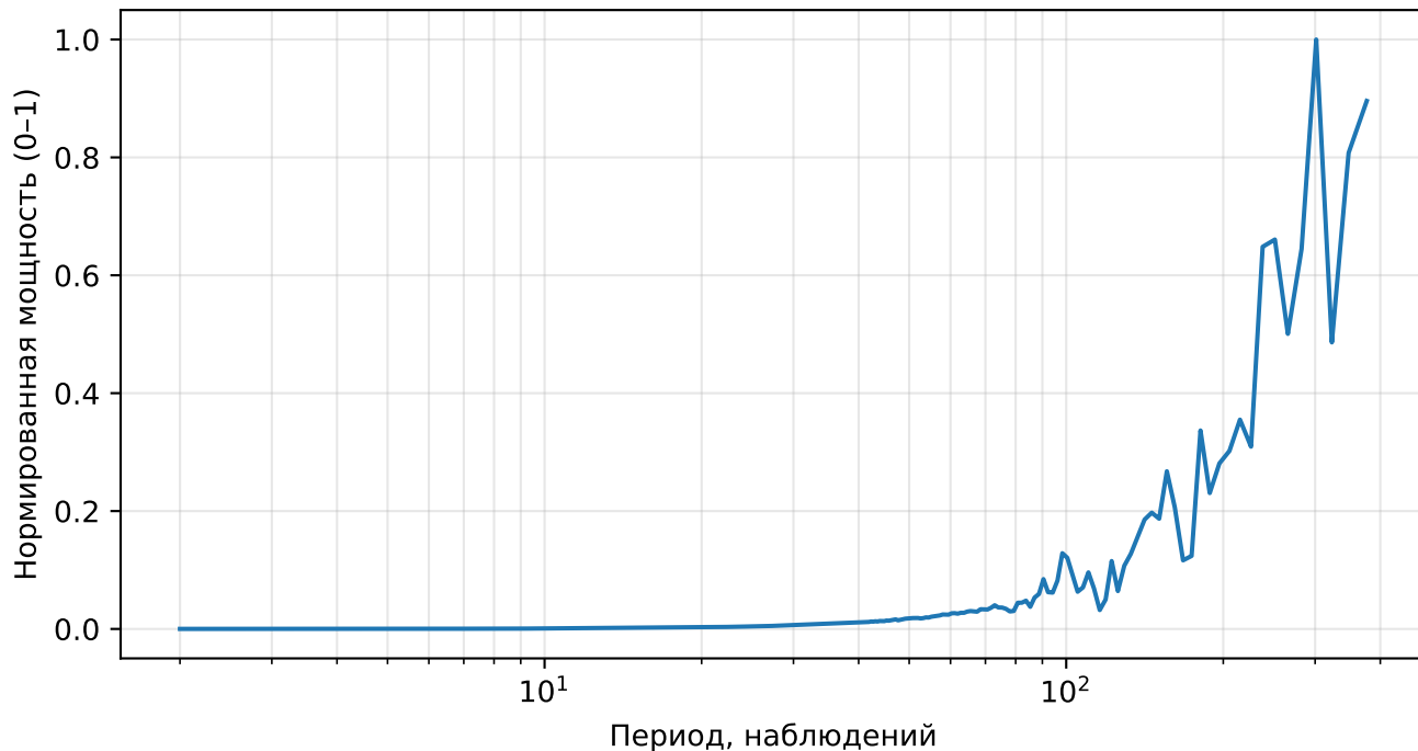
Нормированный спектр реконструкции (AE), price, тикер: RSG
