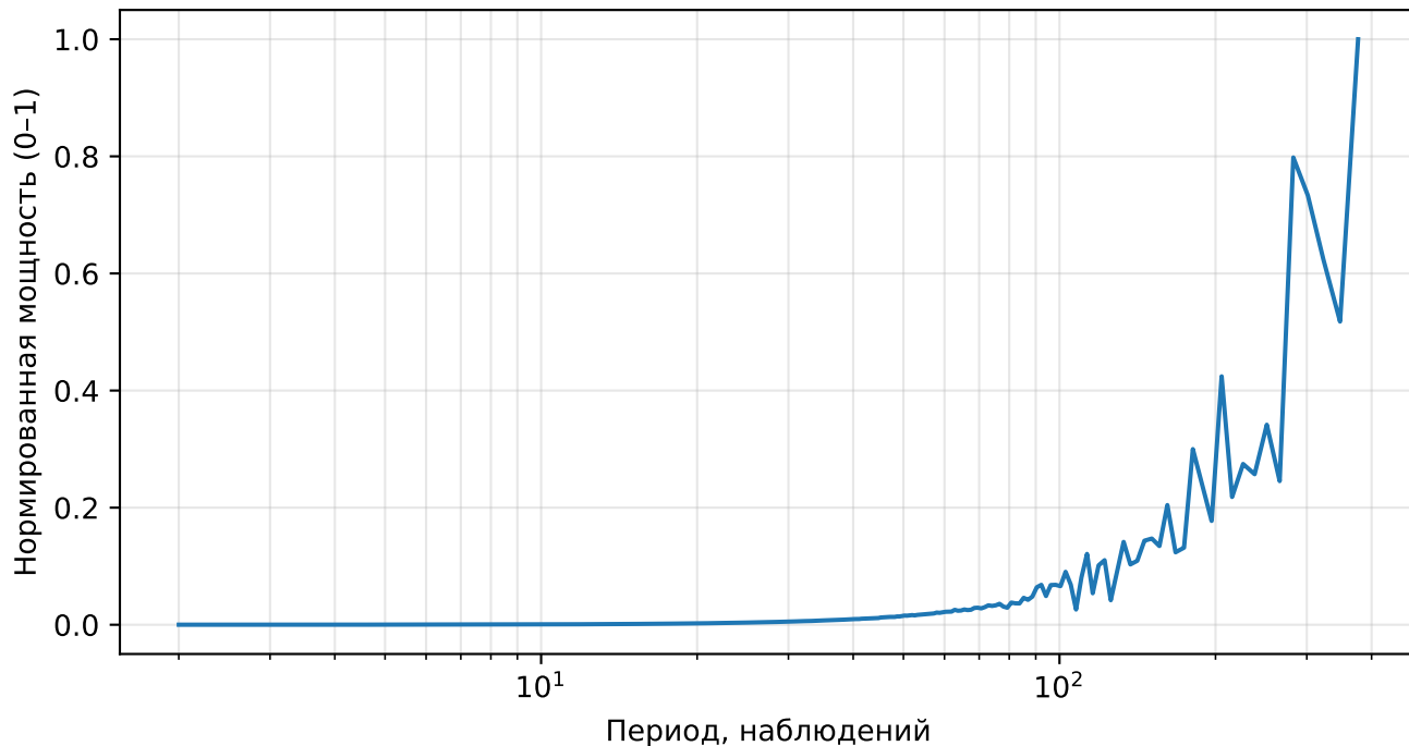
Нормированный спектр реконструкции (AE), price, тикер: TDG
