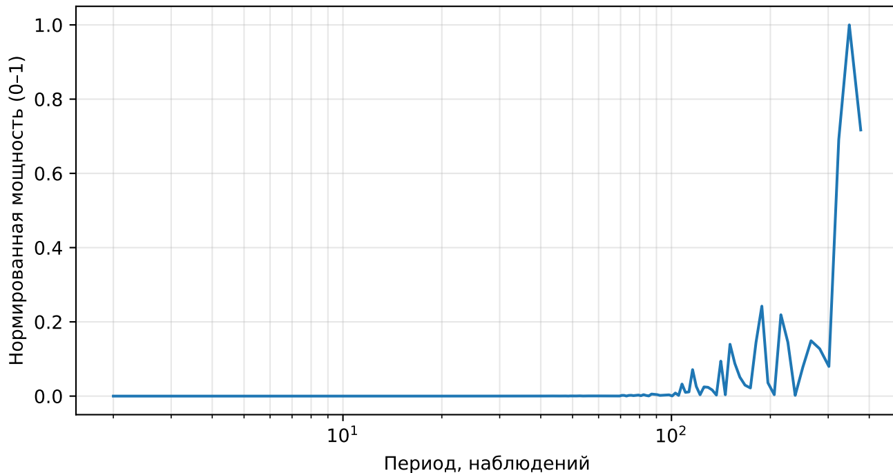
Нормированный спектр реконструкции (AE), price, тикер: SLB
