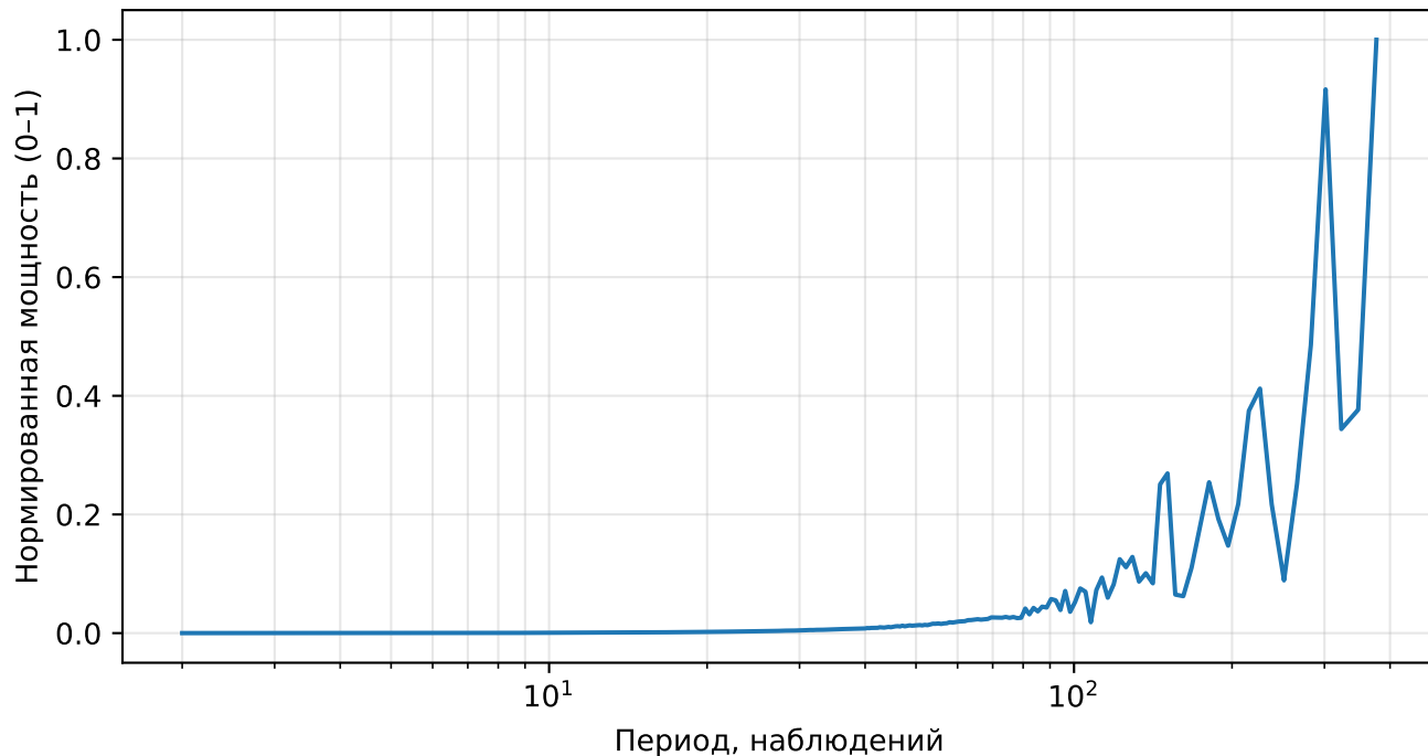
Нормированный спектр реконструкции (AE), price, тикер: TRV
