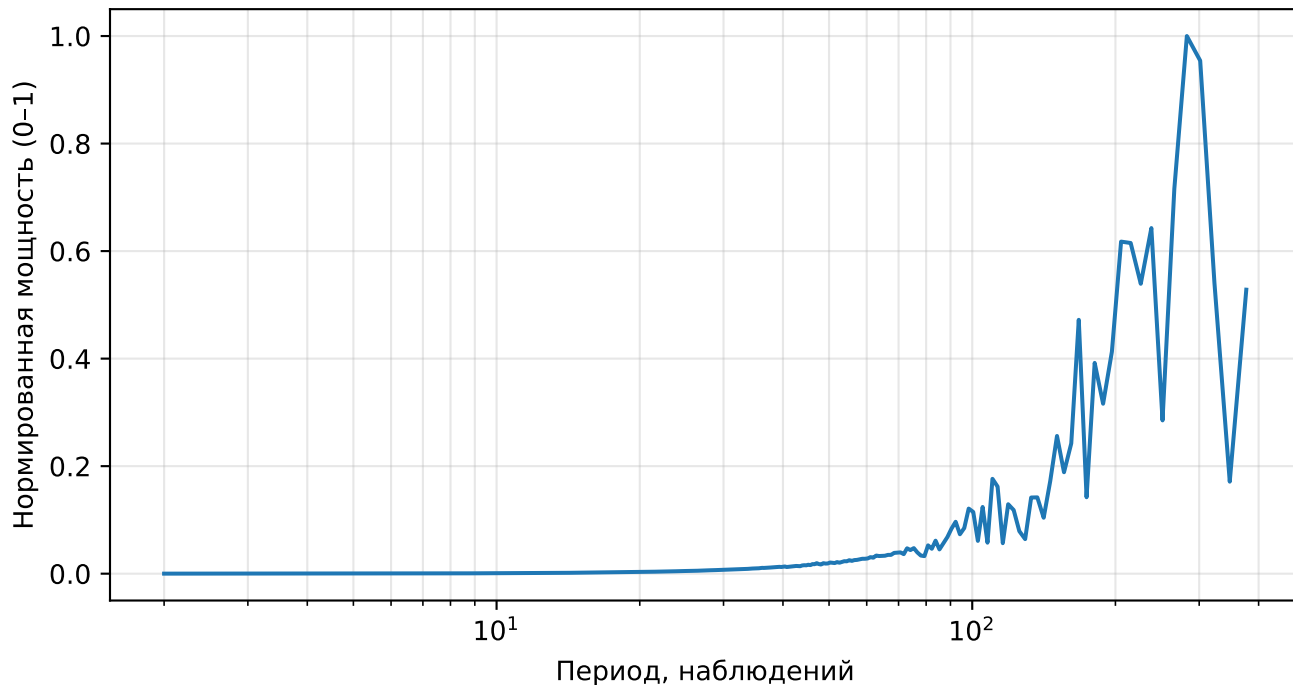
Нормированный спектр реконструкции (AE), price, тикер: ADI
