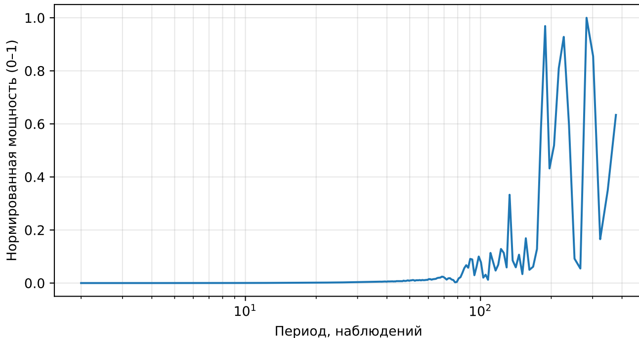
Нормированный спектр реконструкции (AE), price, тикер: F
