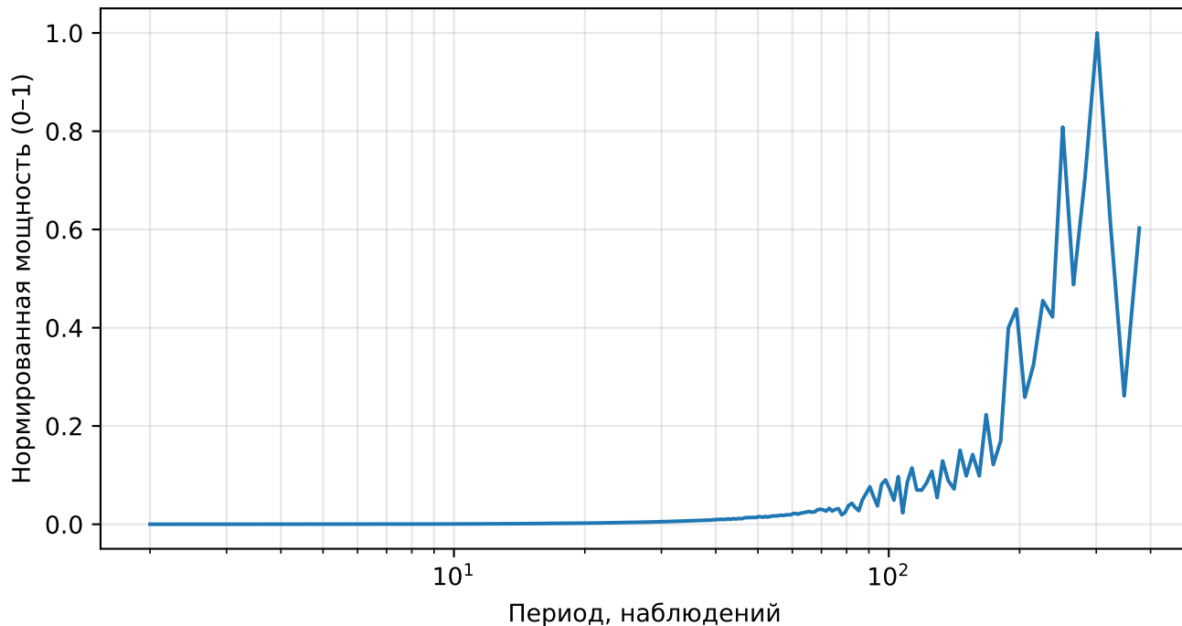
Нормированный спектр реконструкции (AE), price, тикер: ECL
