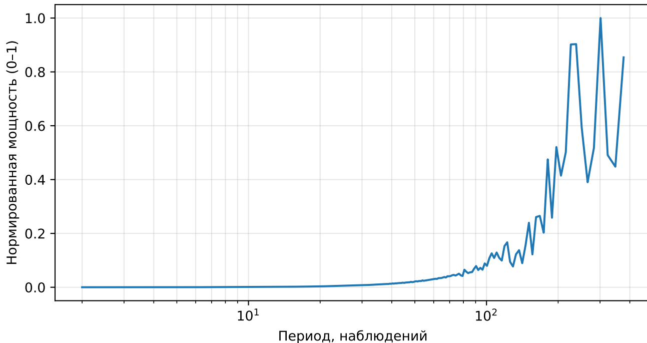
Нормированный спектр реконструкции (AE), price, тикер: TJX
