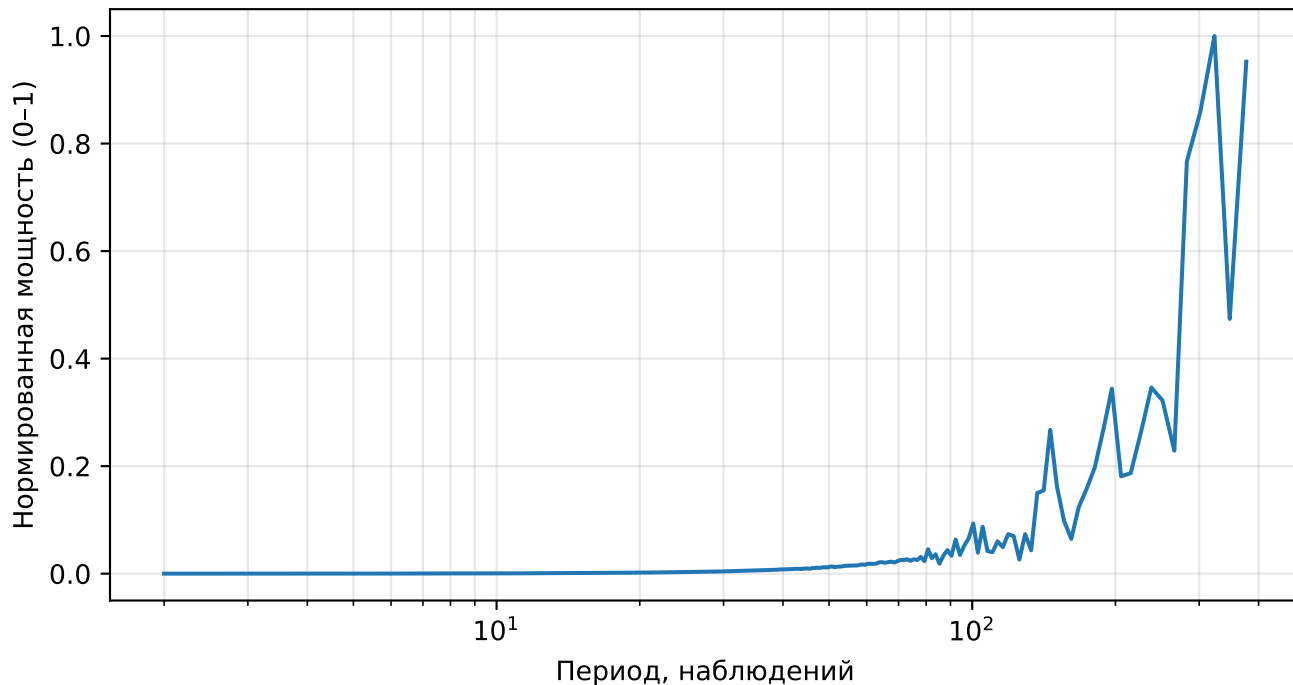
Нормированный спектр реконструкции (AE), price, тикер: ABT
