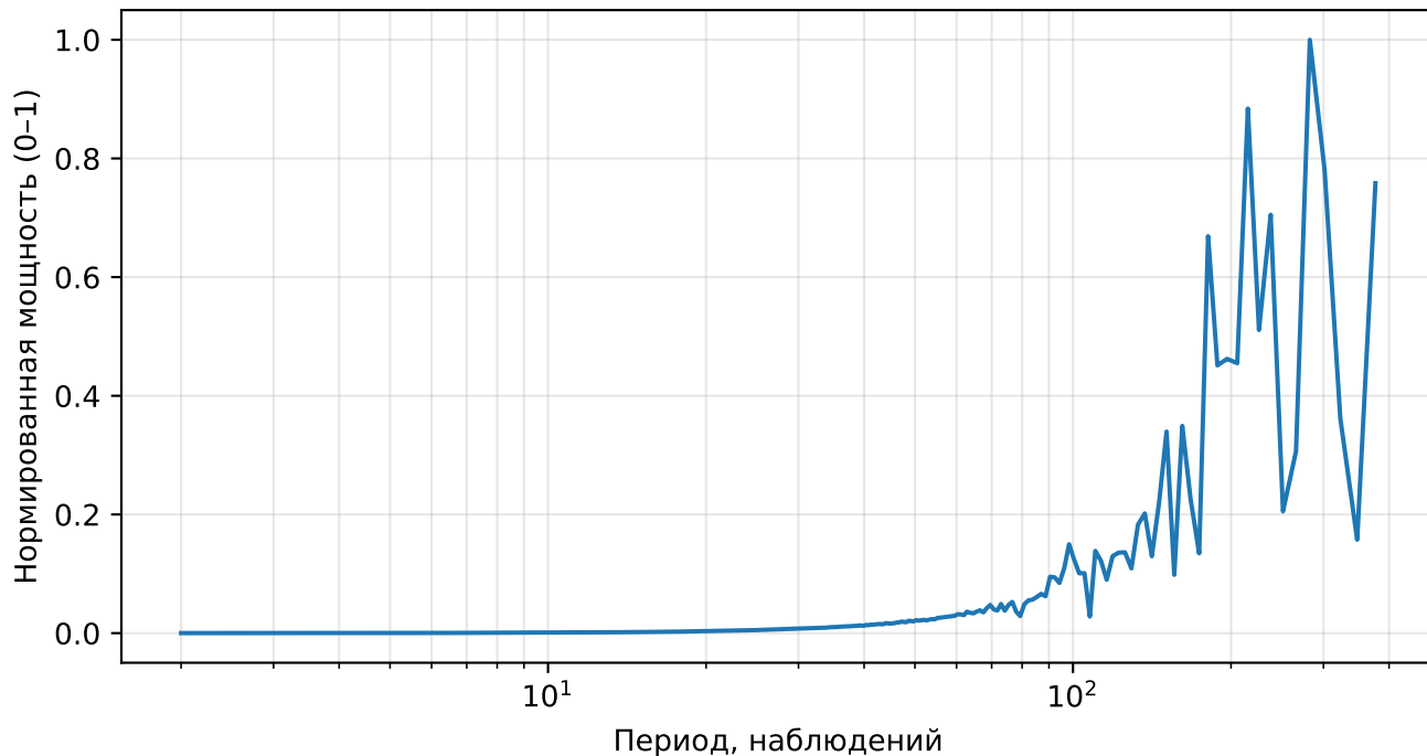
Нормированный спектр реконструкции (AE), price, тикер: PH
