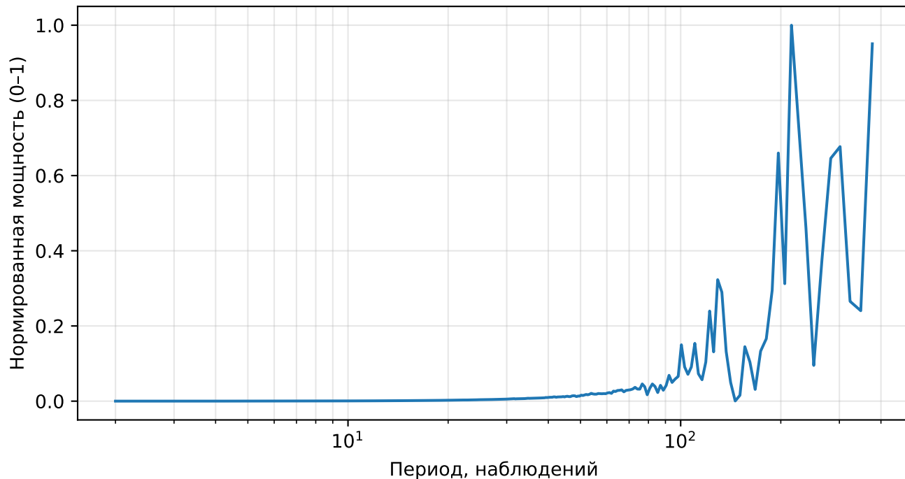
Нормированный спектр реконструкции (AE), price, тикер: CME
