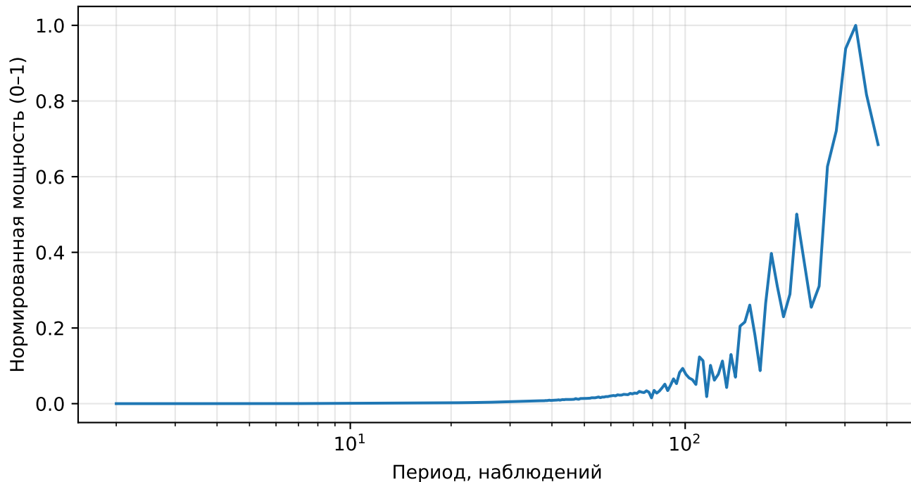
Нормированный спектр реконструкции (AE), price, тикер: LHX
