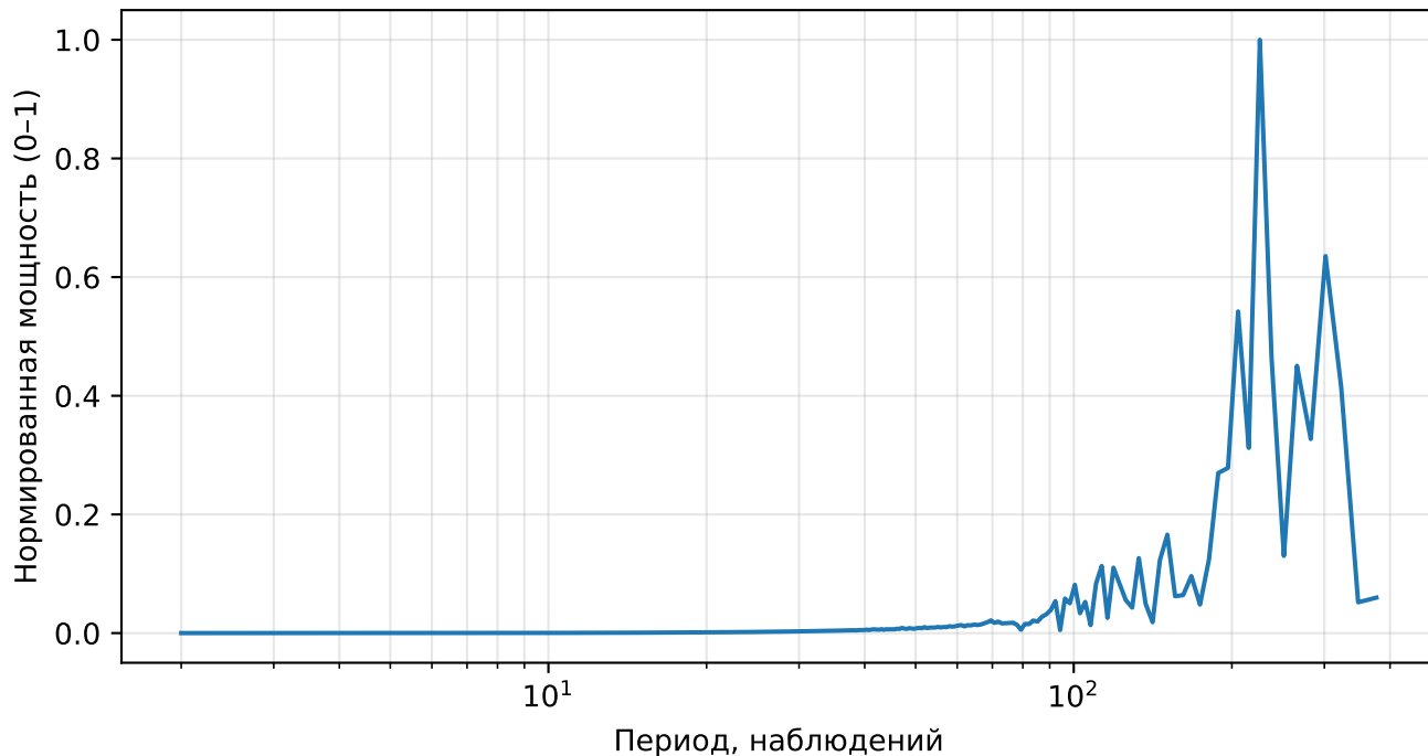
Нормированный спектр реконструкции (AE), price, тикер: ADSK
