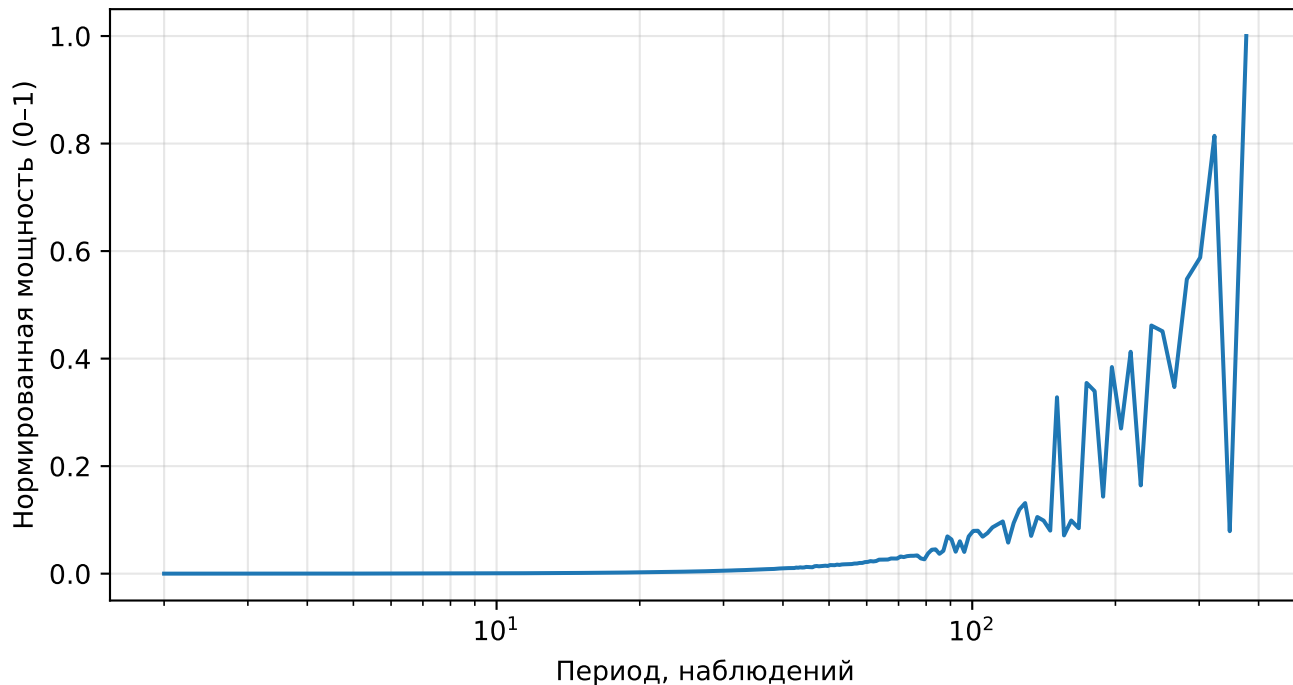
Нормированный спектр реконструкции (AE), price, тикер: WMT
