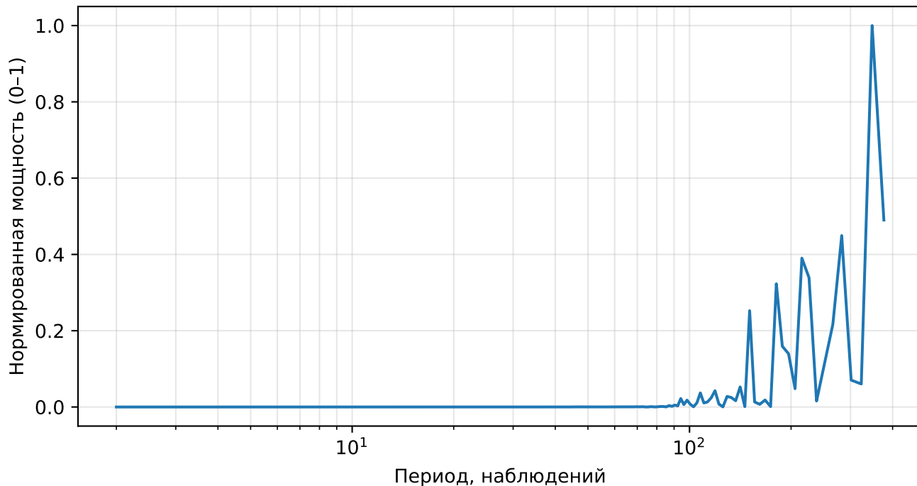
Нормированный спектр реконструкции (AE), price, тикер: FCX
