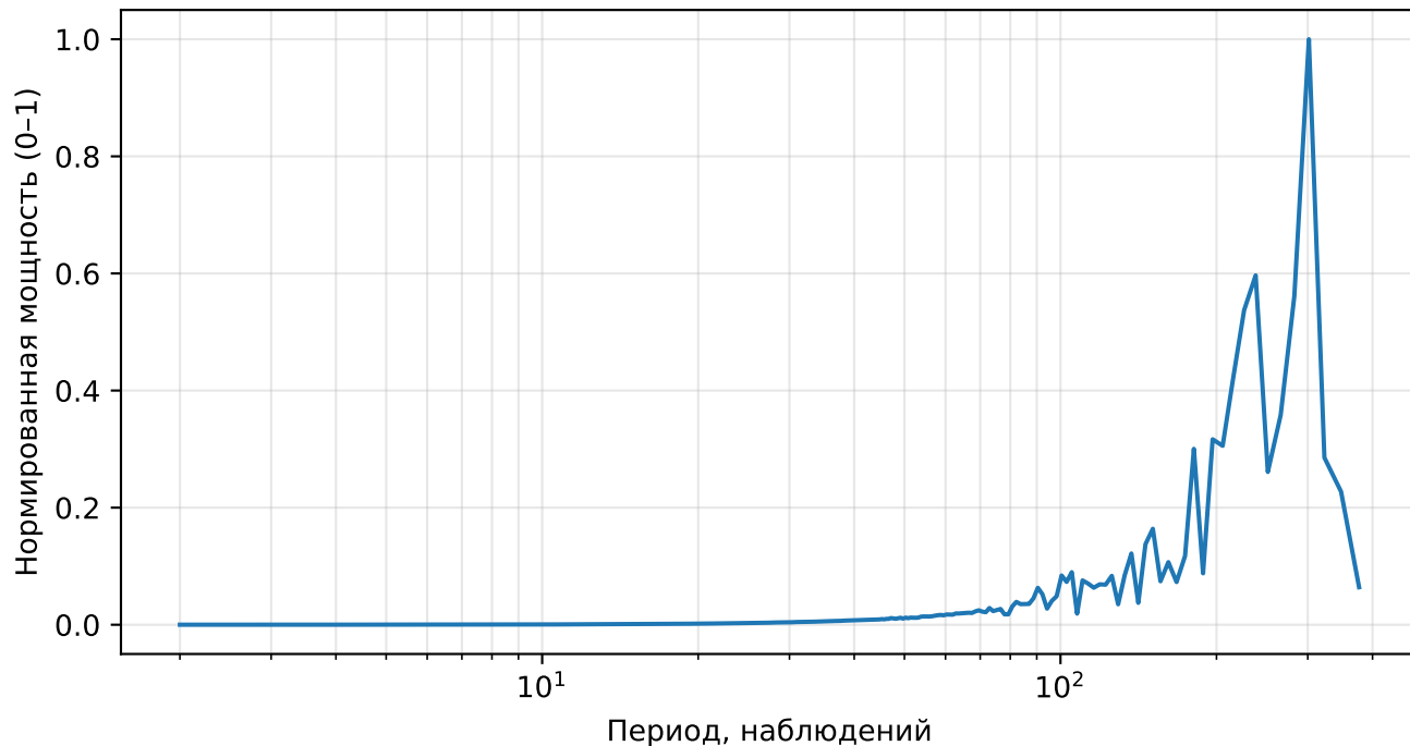
Нормированный спектр реконструкции (AE), price, тикер: CSX
