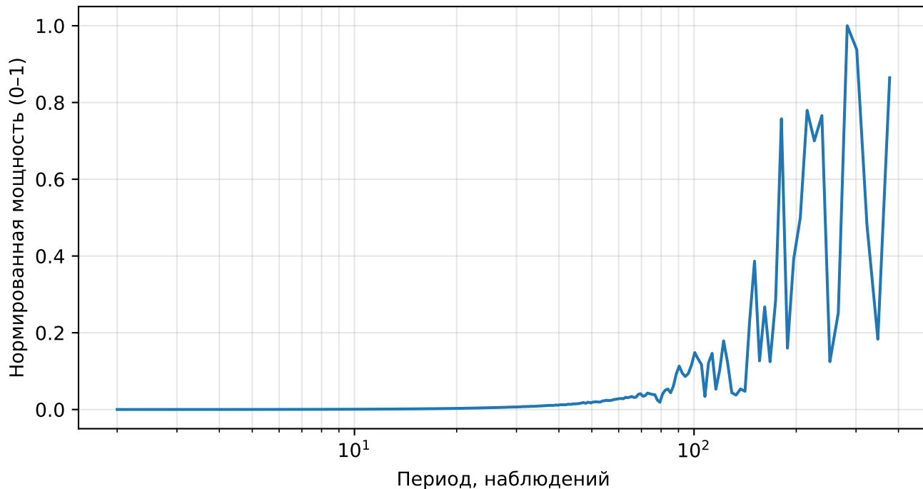
Нормированный спектр реконструкции (AE), price, тикер: HON
