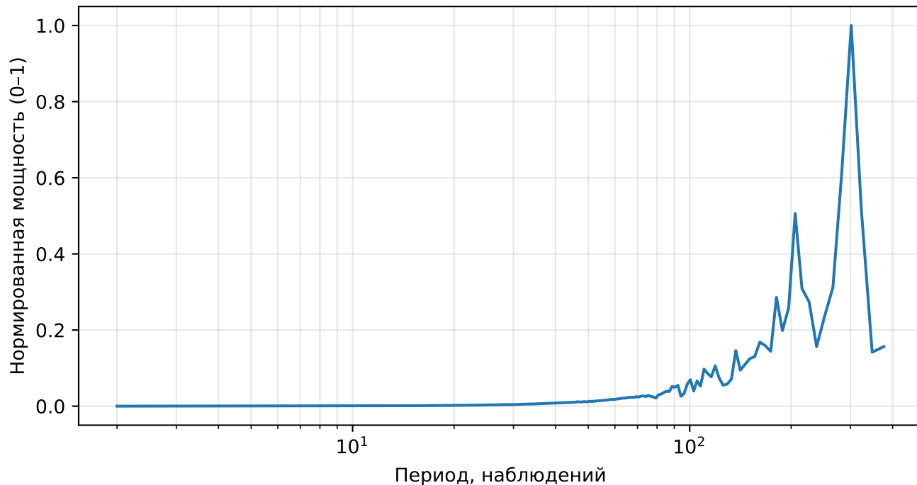
Нормированный спектр реконструкции (AE), price, тикер: NVDA
