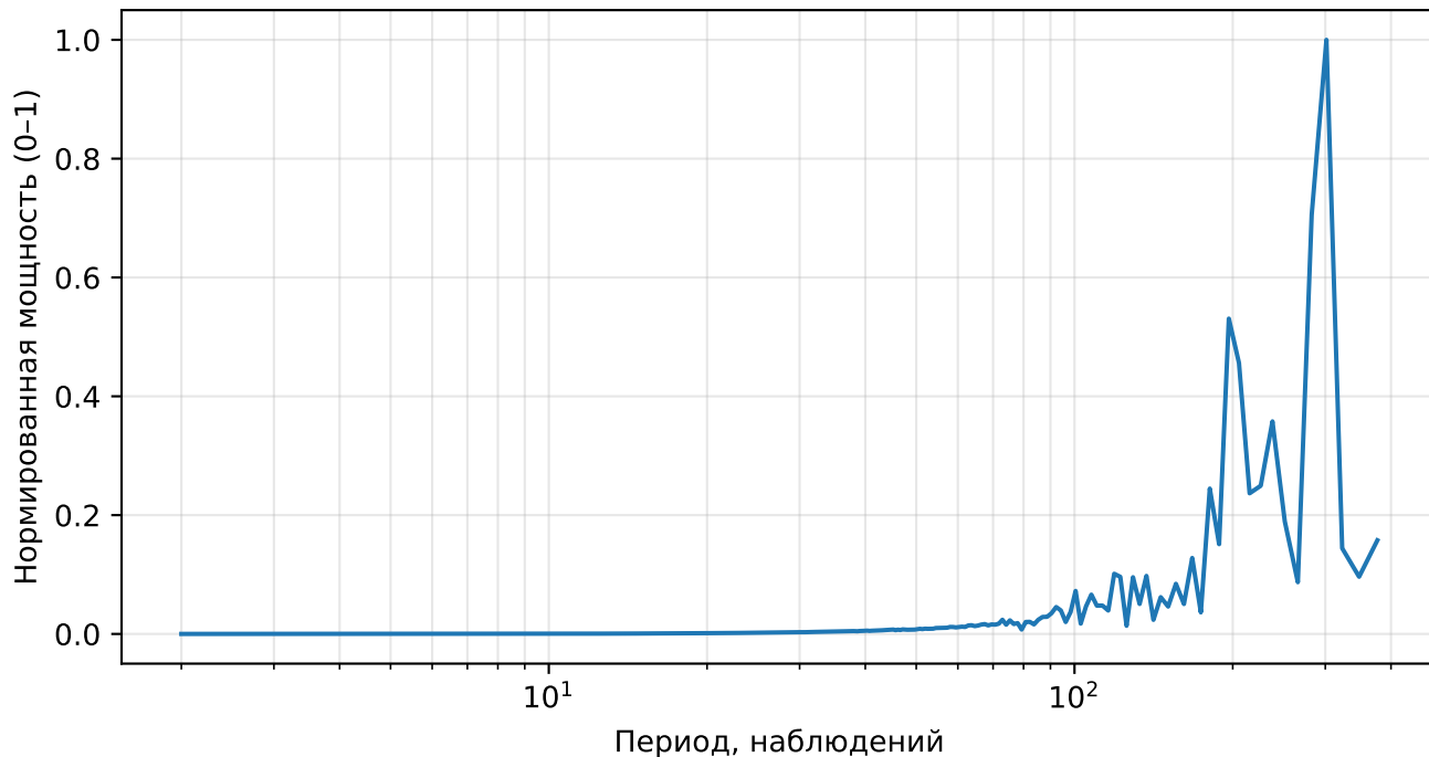
Нормированный спектр реконструкции (AE), price, тикер: AMD
