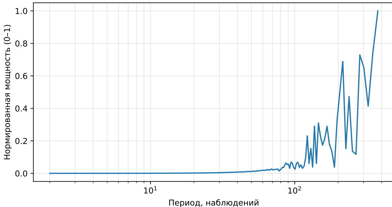
Нормированный спектр реконструкции (AE), price, тикер: T
