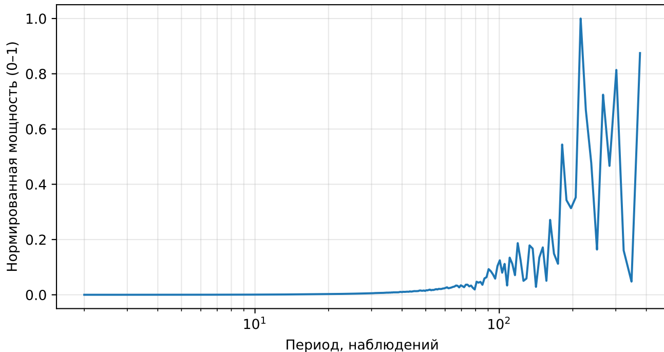
Нормированный спектр реконструкции (AE), price, тикер: CSCO
