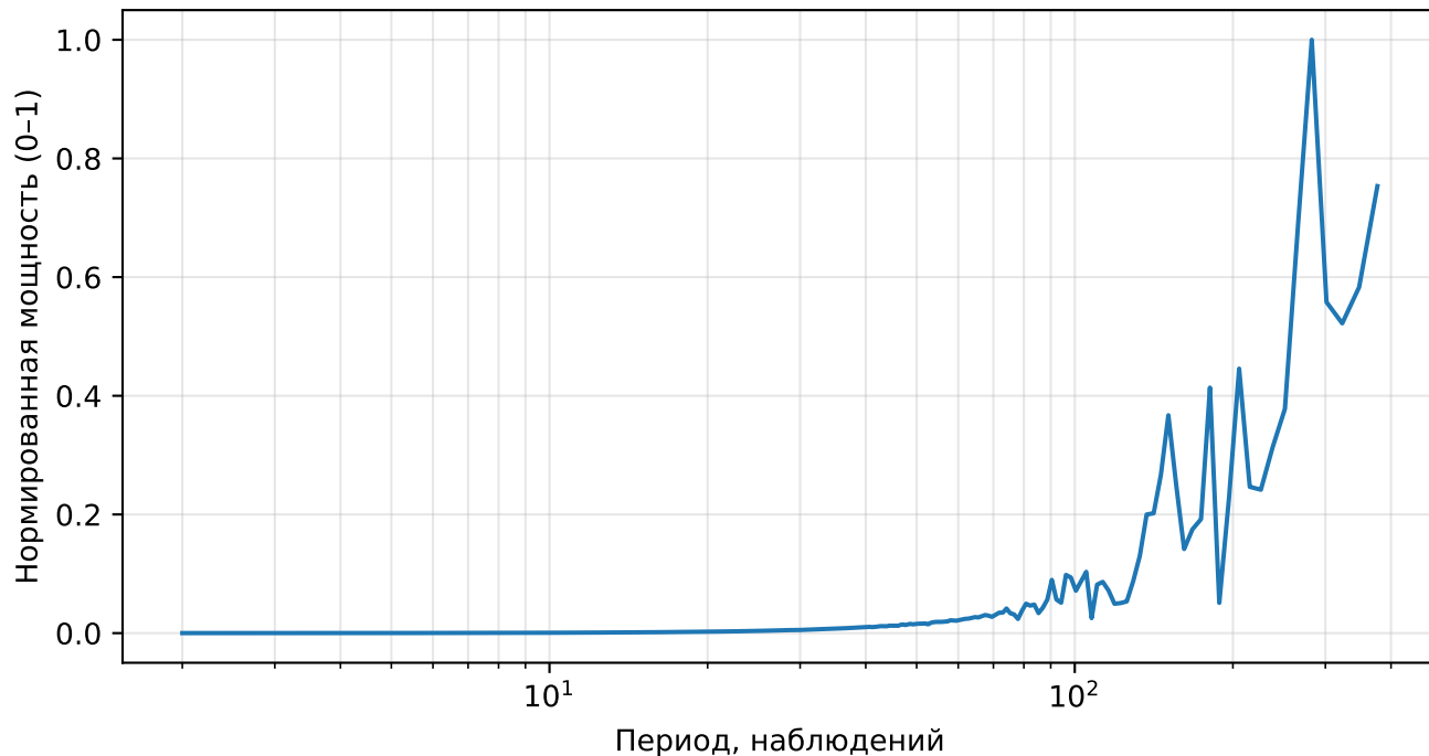
Нормированный спектр реконструкции (AE), price, тикер: AEP
