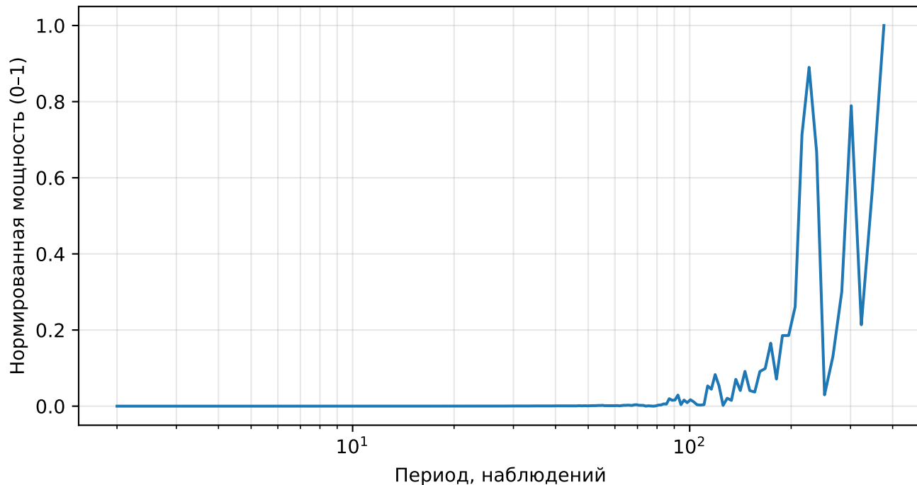
Нормированный спектр реконструкции (AE), price, тикер: ВАС
