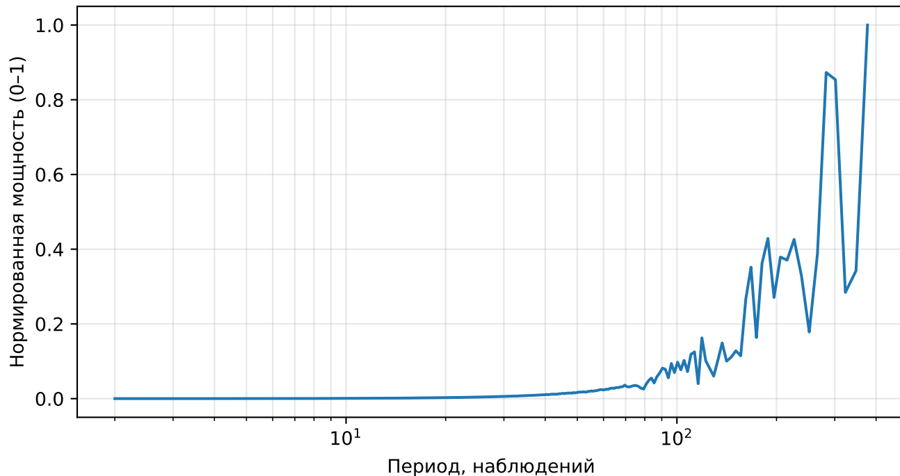
Нормированный спектр реконструкции (AE), price, тикер: LRCX
