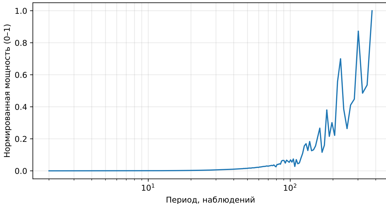
Нормированный спектр реконструкции (AE), price, тикер: PGR
