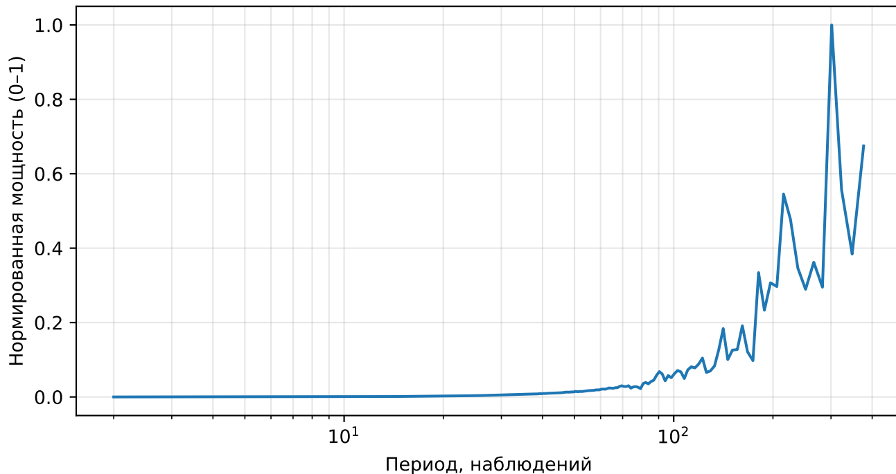
Нормированный спектр реконструкции (AE), price, тикер: HD
