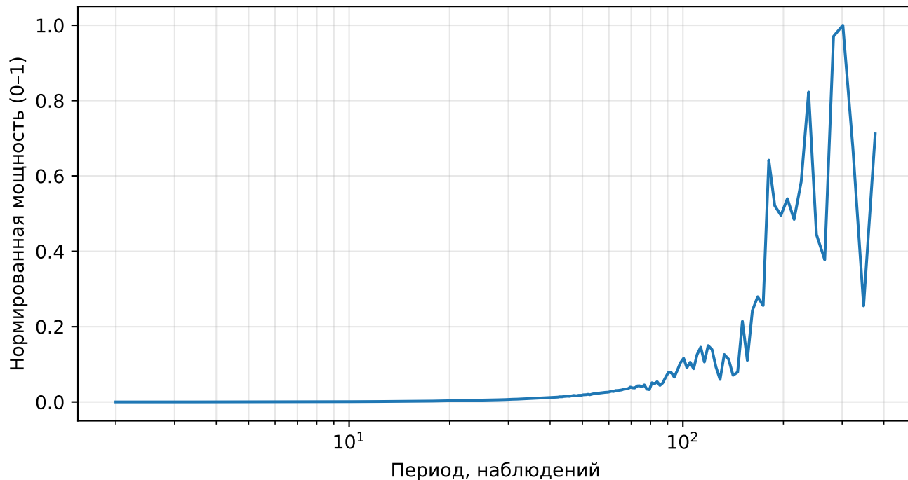
Нормированный спектр реконструкции (AE), price, тикер: APH
