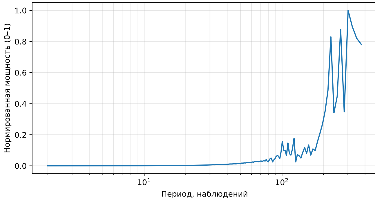
Нормированный спектр реконструкции (AE), price, тикер: NDAQ
