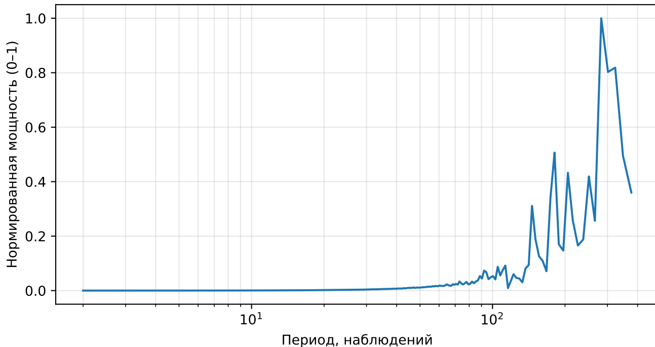
Нормированный спектр реконструкции (AE), price, тикер: MRK
