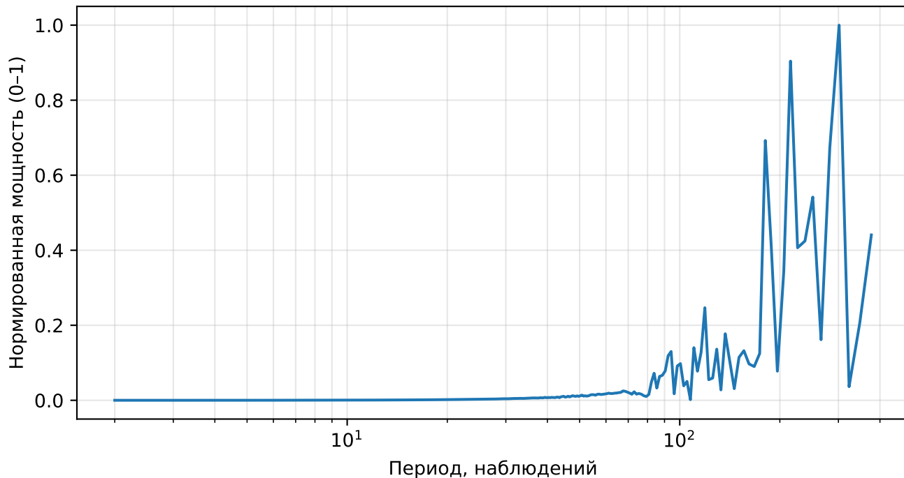
Нормированный спектр реконструкции (AE), price, тикер: UPS
