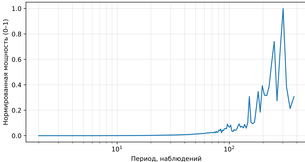
Нормированный спектр реконструкции (AE), price, тикер: PEP
