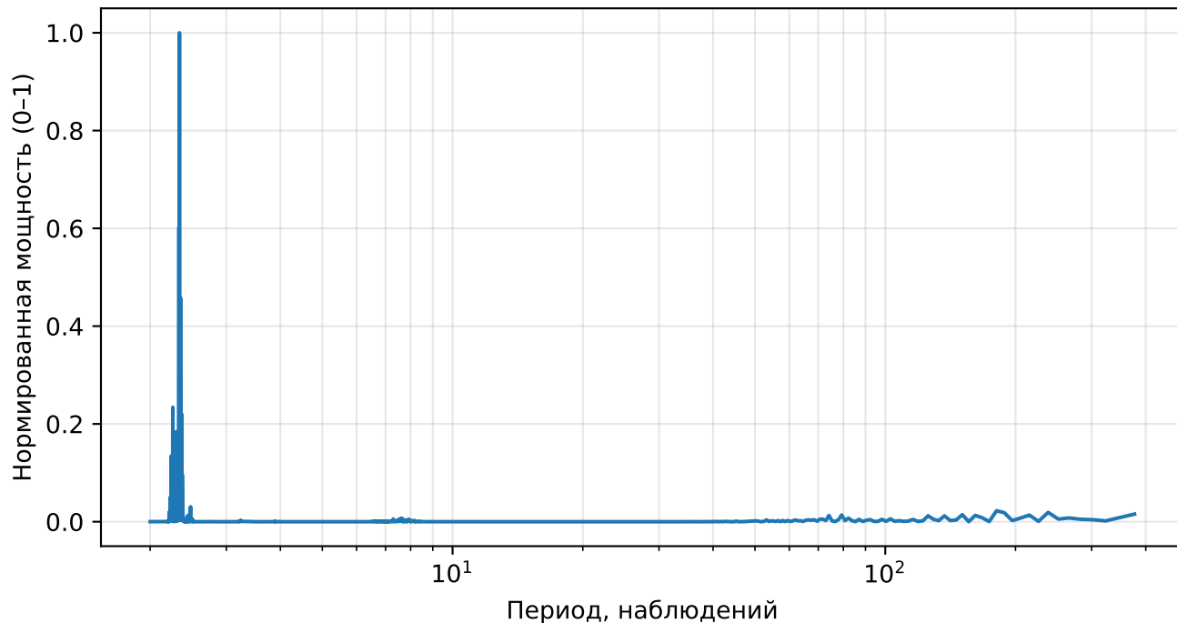
Нормированный спектр реконструкции (AE), returns, тикер: MS
