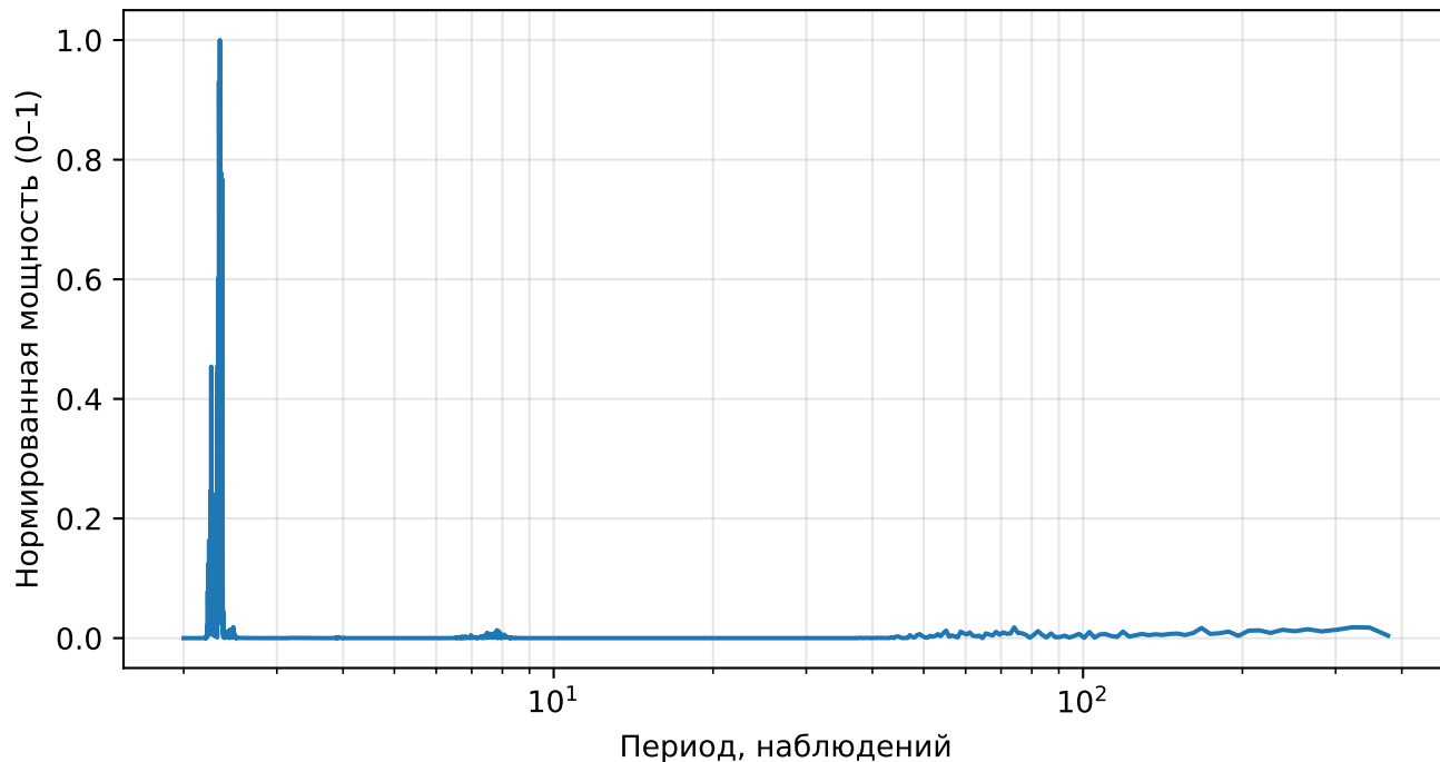
Нормированный спектр реконструкции (AE), returns, тикер: PEP
