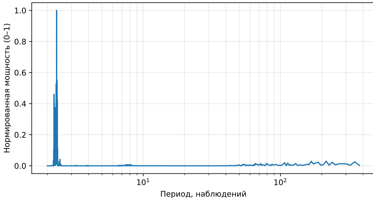
Нормированный спектр реконструкции (AE), returns, тикер: MMC
