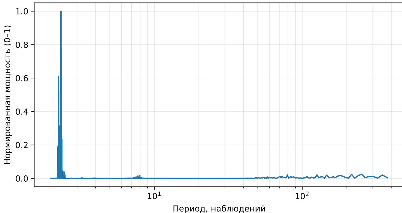
Нормированный спектр реконструкции (AE), returns, тикер: AXP
