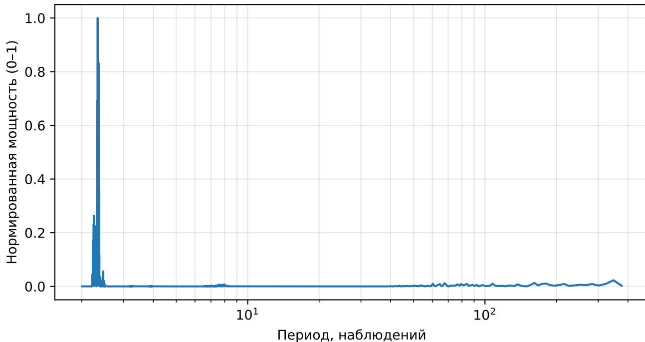
Нормированный спектр реконструкции (AE), returns, тикер: NKE
