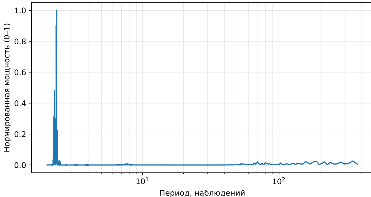
Нормированный спектр реконструкции (AE), returns, тикер: EMR
