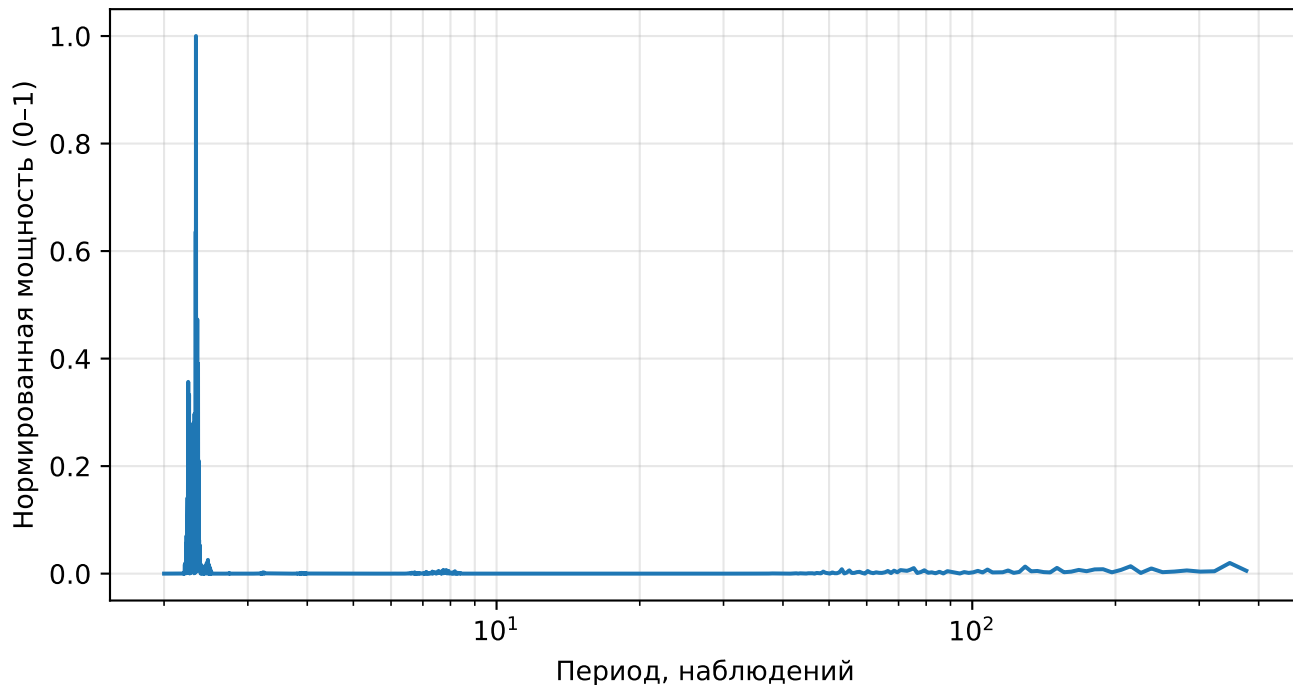
Нормированный спектр реконструкции (AE), returns, тикер: CMCSA
