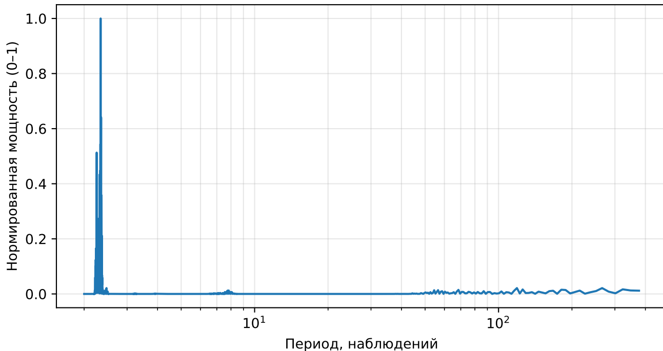
Нормированный спектр реконструкции (AE), returns, тикер: UNH
