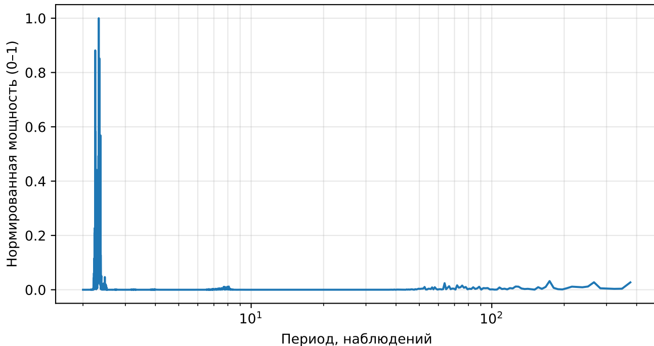
Нормированный спектр реконструкции (AE), returns, тикер: MNST
