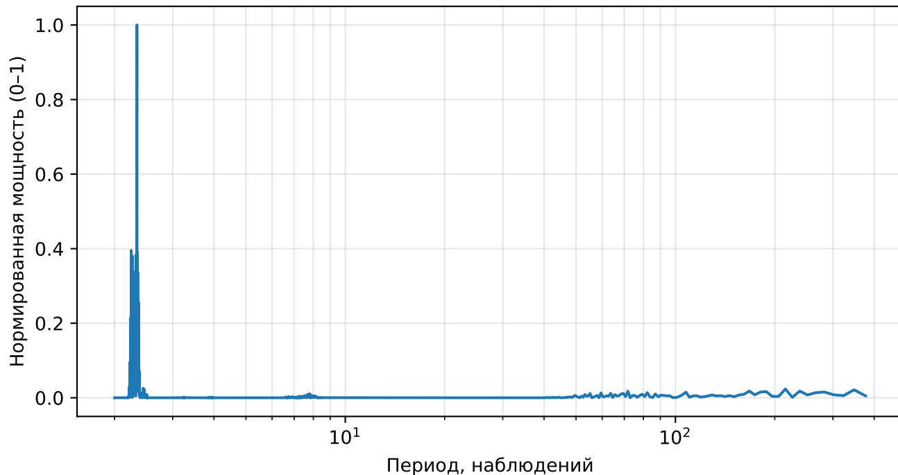
Нормированный спектр реконструкции (AE), returns, тикер: AJG
