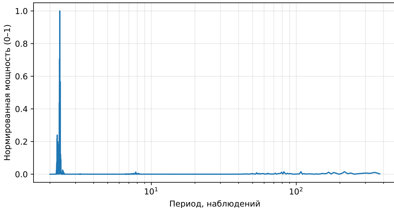
Нормированный спектр реконструкции (AE), returns, тикер: PGR
