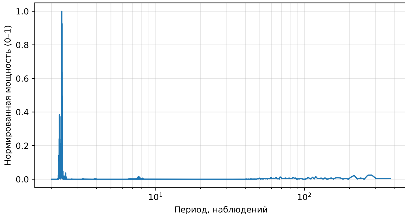
Нормированный спектр реконструкции (AE), returns, тикер: CVS
