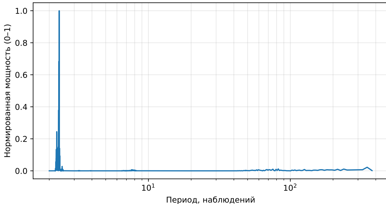
Нормированный спектр реконструкции (AE), returns, тикер: IBM
