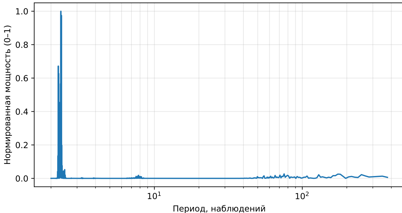
Нормированный спектр реконструкции (AE), returns, тикер: SBUX
