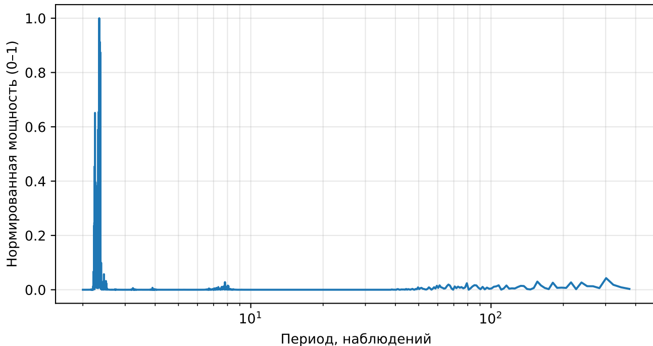
Нормированный спектр реконструкции (AE), returns, тикер: DHR
