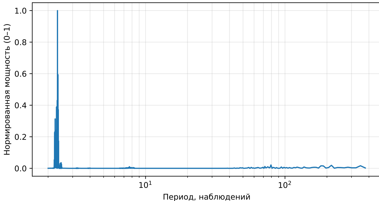
Нормированный спектр реконструкции (AE), returns, тикер: PCAR
