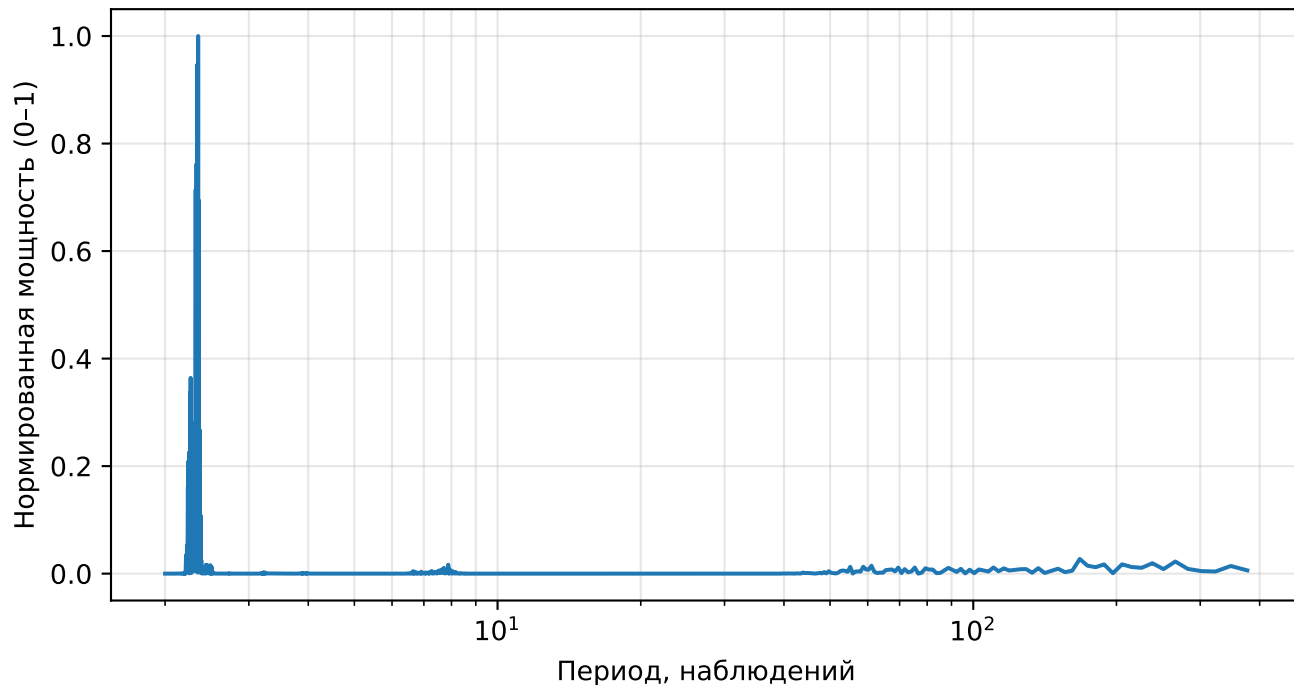
Нормированный спектр реконструкции (AE), returns, тикер: SPGI
