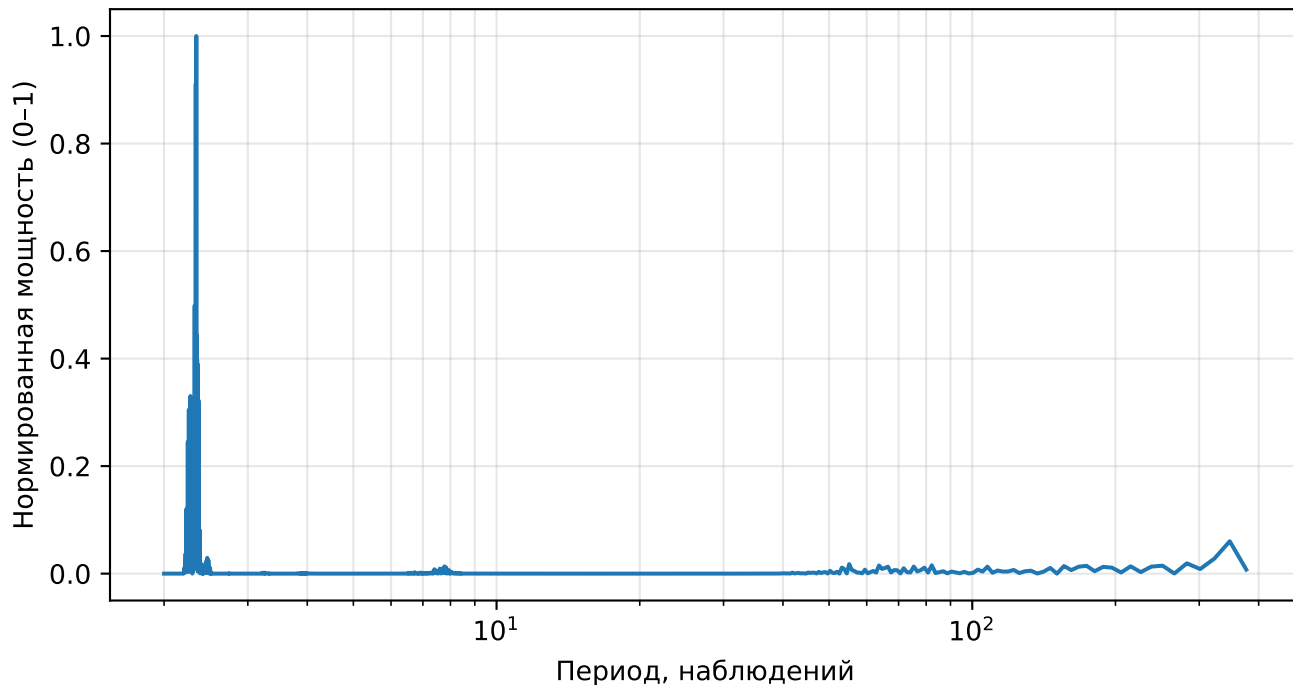
Нормированный спектр реконструкции (AE), returns, тикер: AFL
