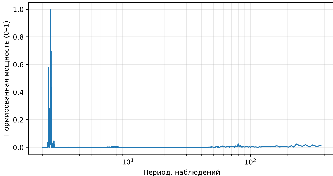
Нормированный спектр реконструкции (AE), returns, тикер: MSI
