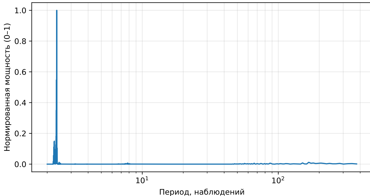
Нормированный спектр реконструкции (AE), returns, тикер: CRM
