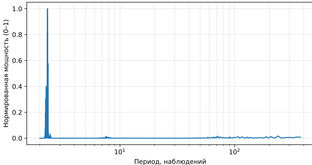
Нормированный спектр реконструкции (AE), returns, тикер: MU
