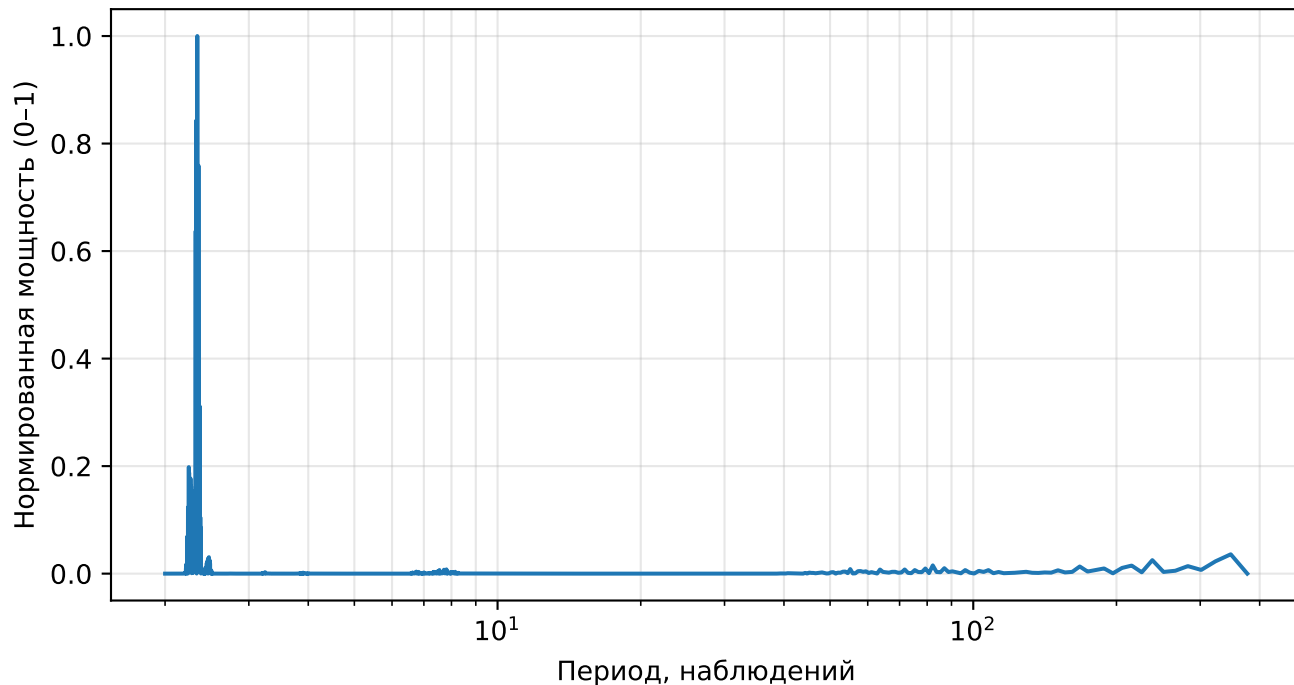
Нормированный спектр реконструкции (AE), returns, тикер: ALL
