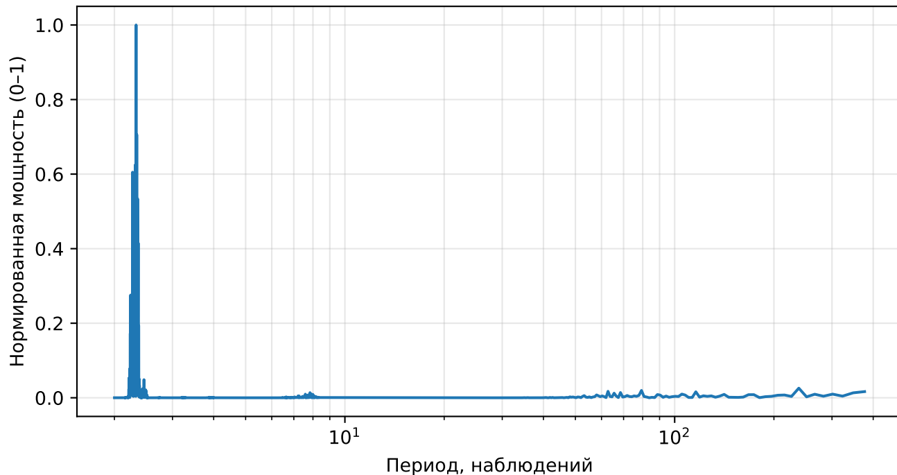
Нормированный спектр реконструкции (AE), returns, тикер: AMD
