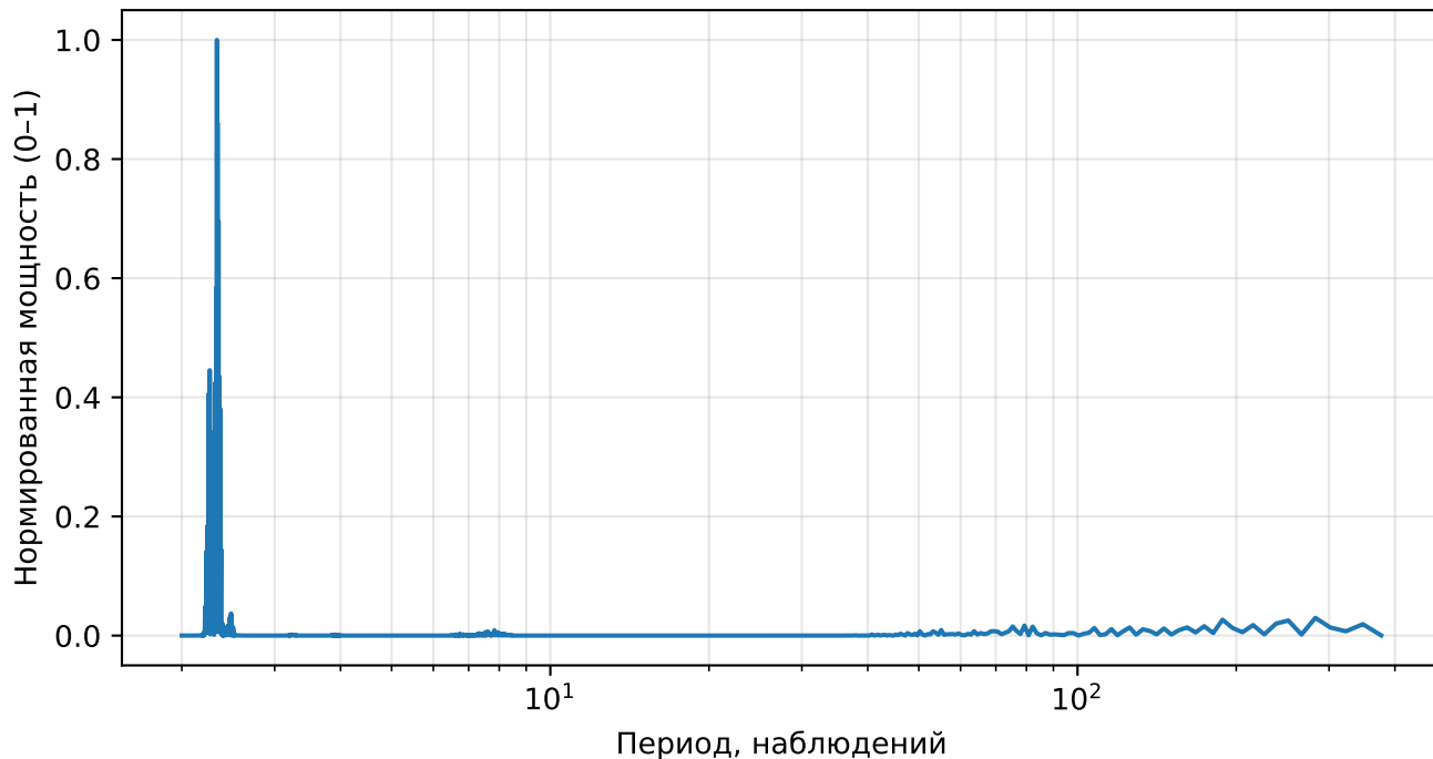
Нормированный спектр реконструкции (AE), returns, тикер: WFC
