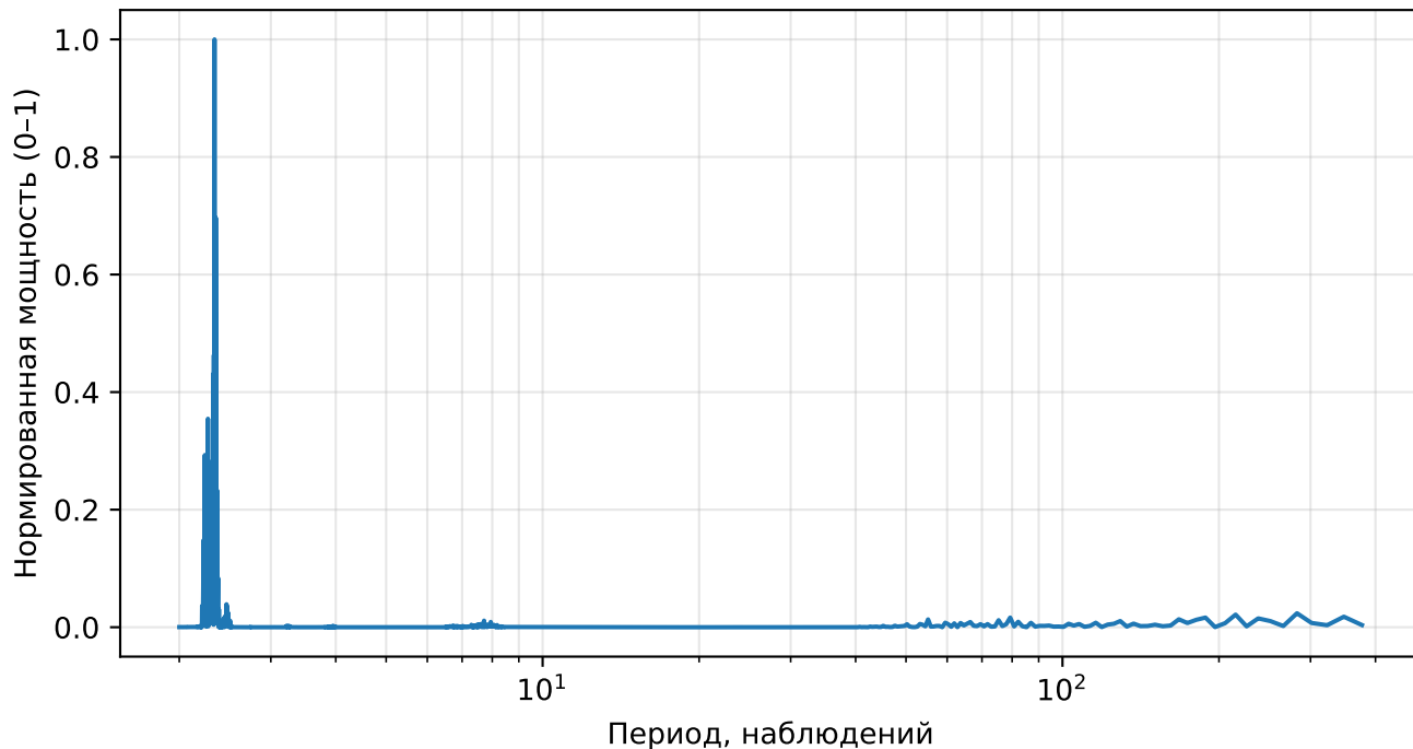
Нормированный спектр реконструкции (AE), returns, тикер: BLK
