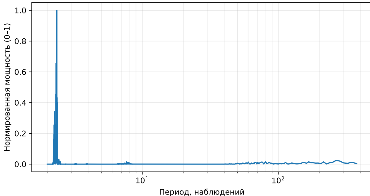
Нормированный спектр реконструкции (AE), returns, тикер: ABT
