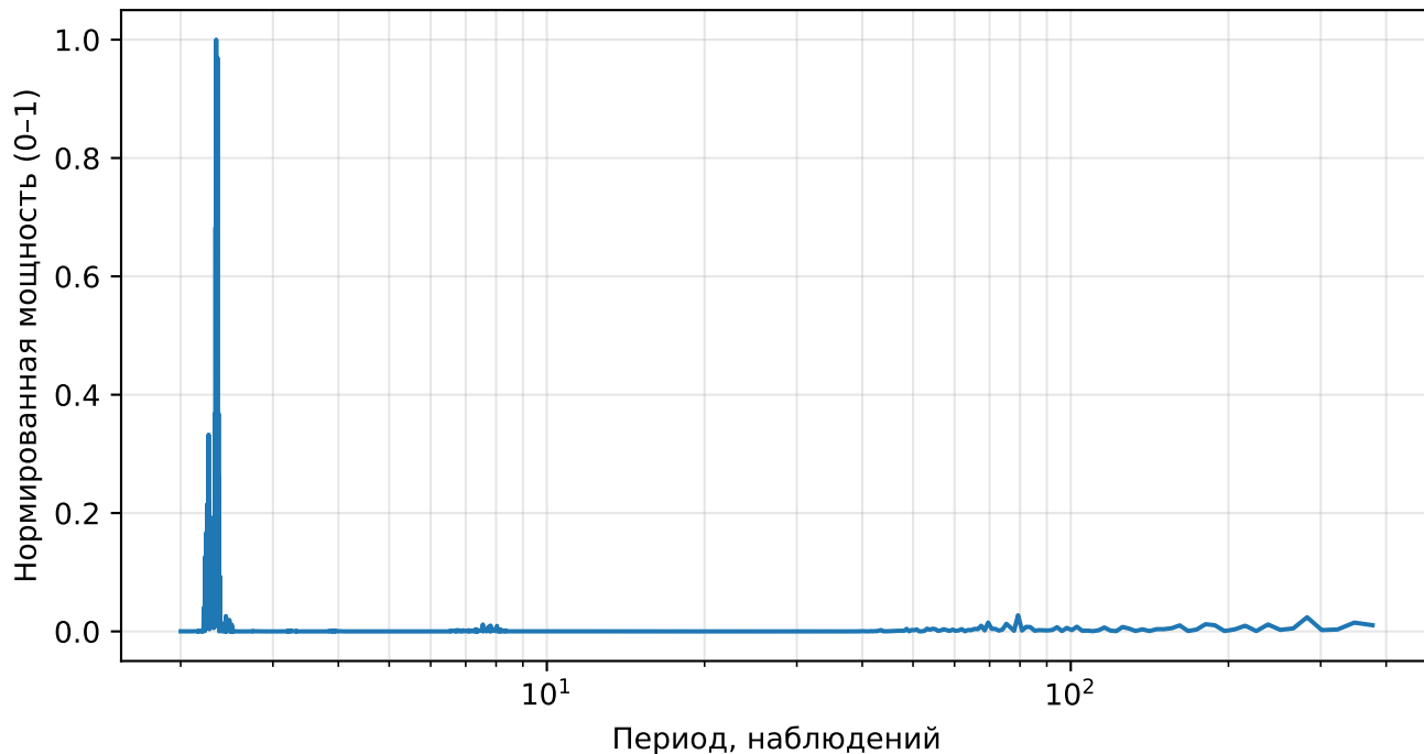
Нормированный спектр реконструкции (AE), returns, тикер: CAT
