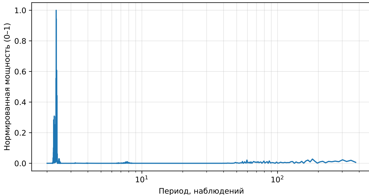
Нормированный спектр реконструкции (AE), returns, тикер: HD
