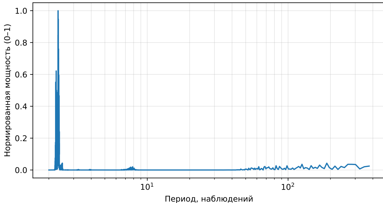
Нормированный спектр реконструкции (AE), returns, тикер: ELV
