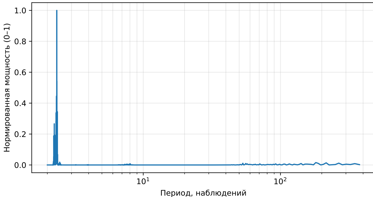
Нормированный спектр реконструкции (AE), returns, тикер: BDX
