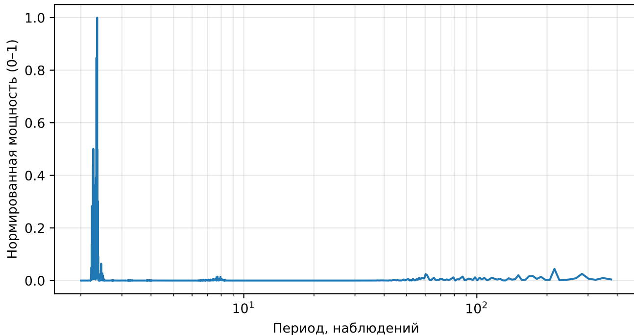
Нормированный спектр реконструкции (AE), returns, тикер: ВМУ
