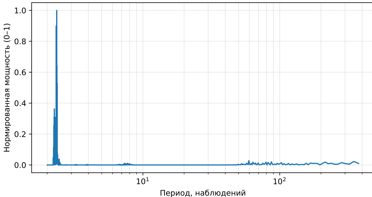
Нормированный спектр реконструкции (АЕ), returns, тикер: ВХ
