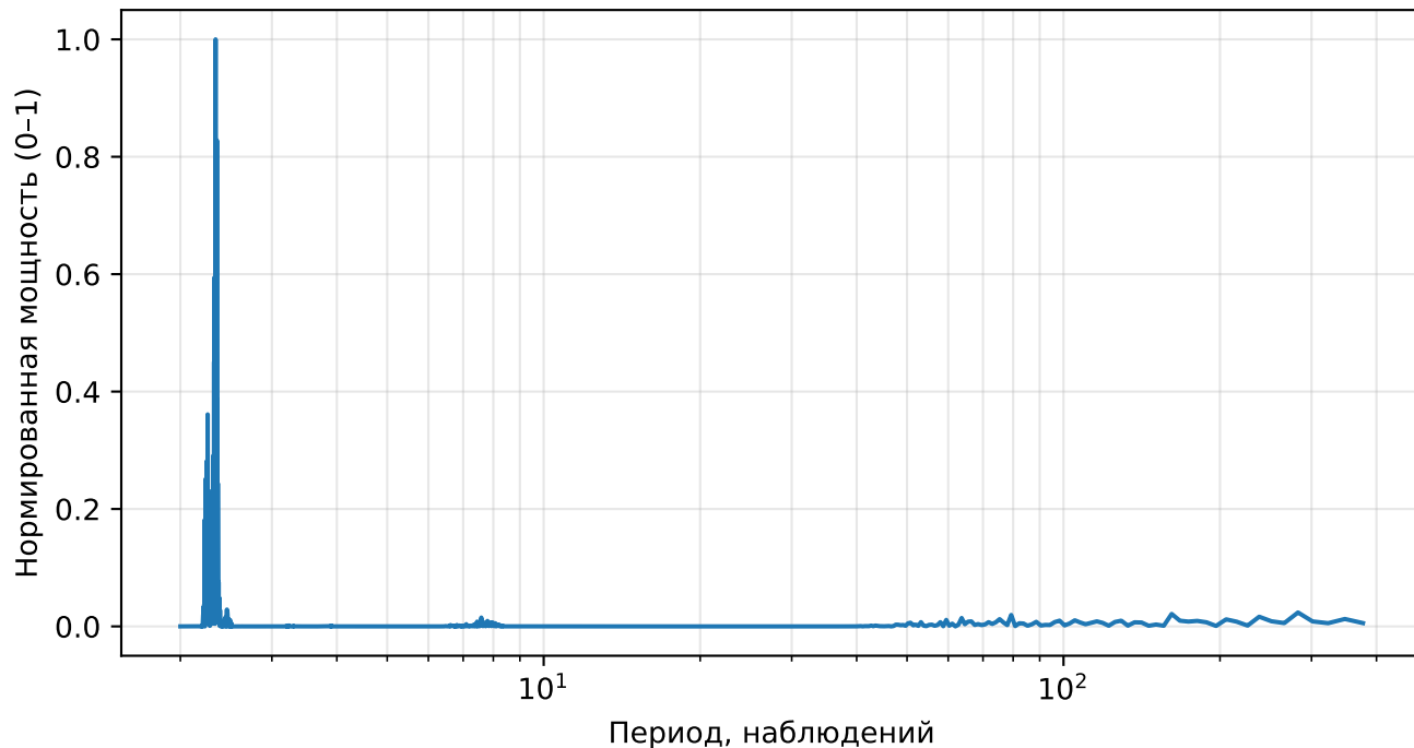
Нормированный спектр реконструкции (AE), returns, тикер: АМАТ
