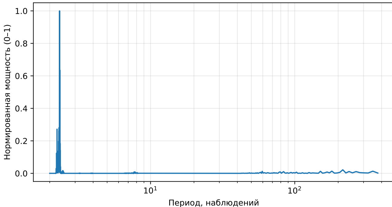
Нормированный спектр реконструкции (AE), returns, тикер: EQIX
