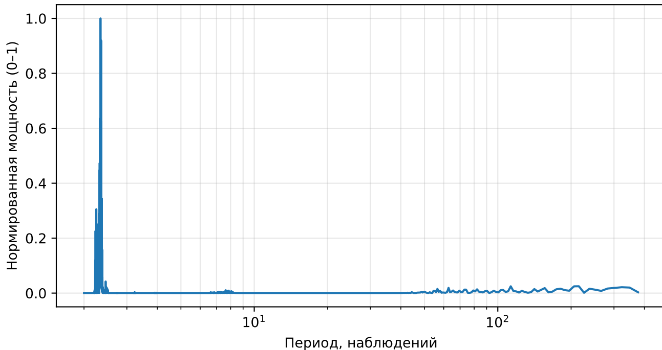
Нормированный спектр реконструкции (AE), returns, тикер: SRE
