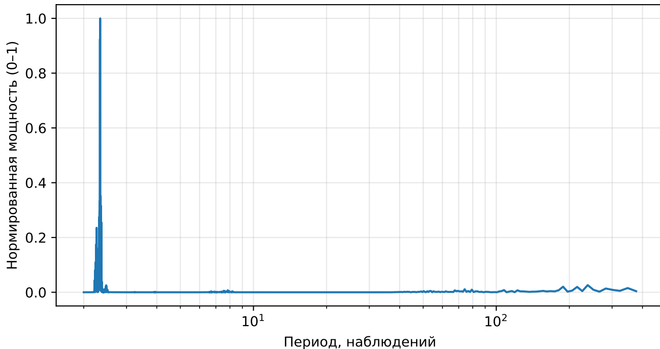
Нормированный спектр реконструкции (АЕ), returns, тикер: С
