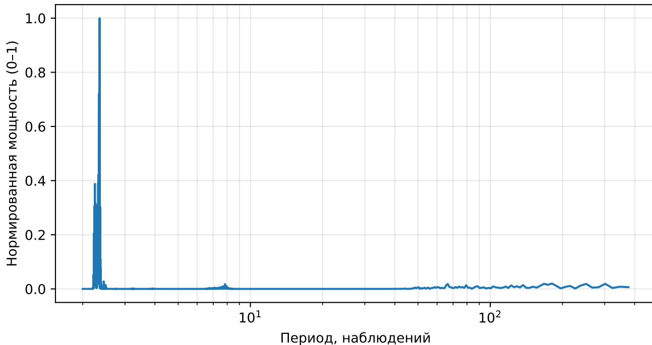
Нормированный спектр реконструкции (AE), returns, тикер: MSFT
