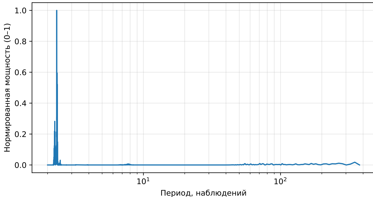
Нормированный спектр реконструкции (АЕ), returns, тикер: JNJ
