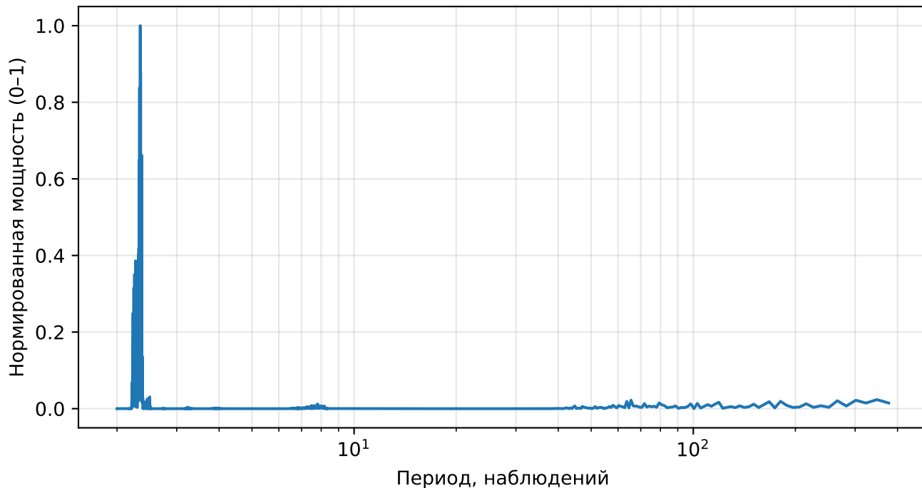
Нормированный спектр реконструкции (АЕ), returns, тикер: NOC
