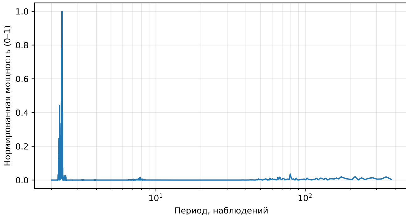
Нормированный спектр реконструкции (AE), returns, тикер: ITW
