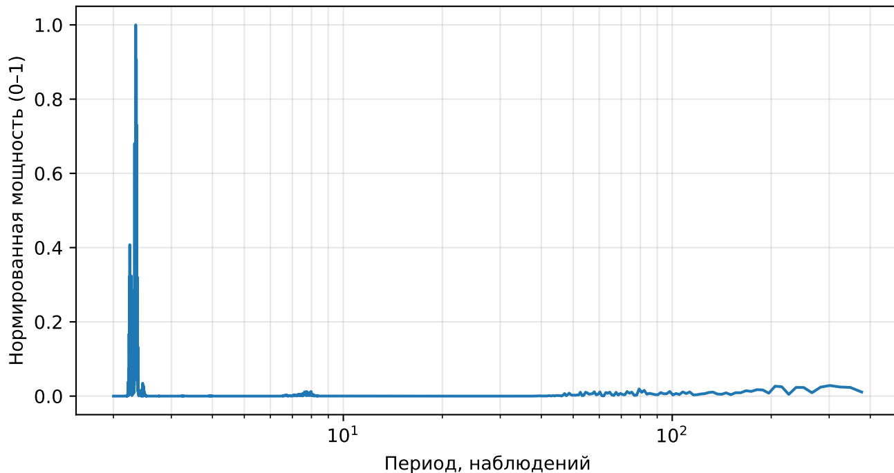
Нормированный спектр реконструкции (AE), returns, тикер: SO
