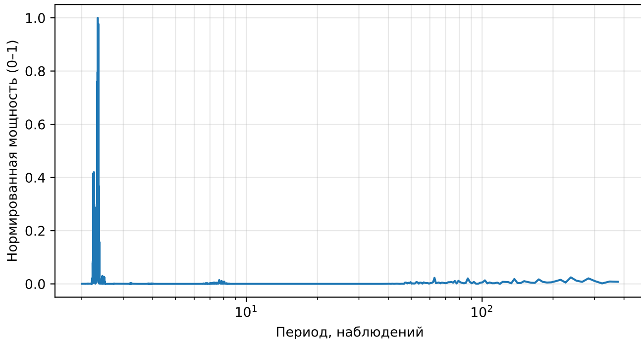
Нормированный спектр реконструкции (AE), returns, тикер: ORCL
