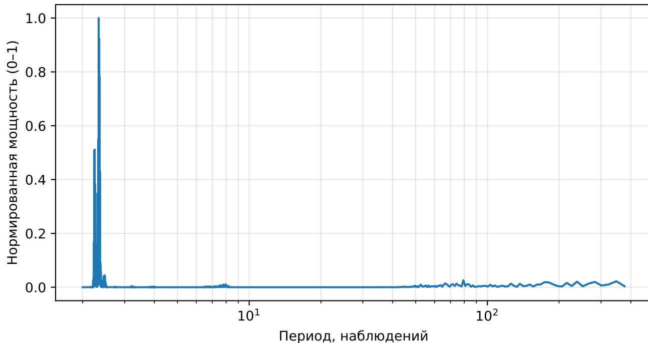
Нормированный спектр реконструкции (AE), returns, тикер: HON
