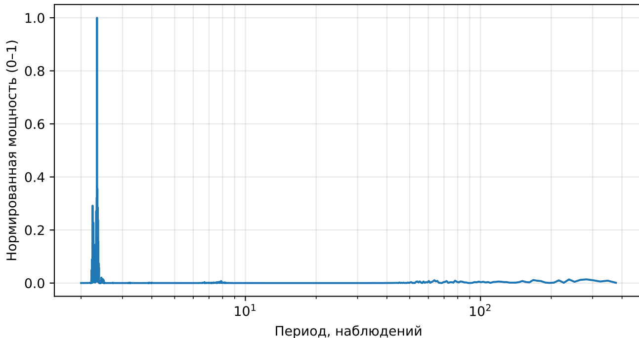
Нормированный спектр реконструкции (AE), returns, тикер: SHW
