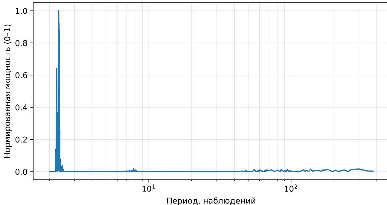
Нормированный спектр реконструкции (AE), returns, тикер: MO
