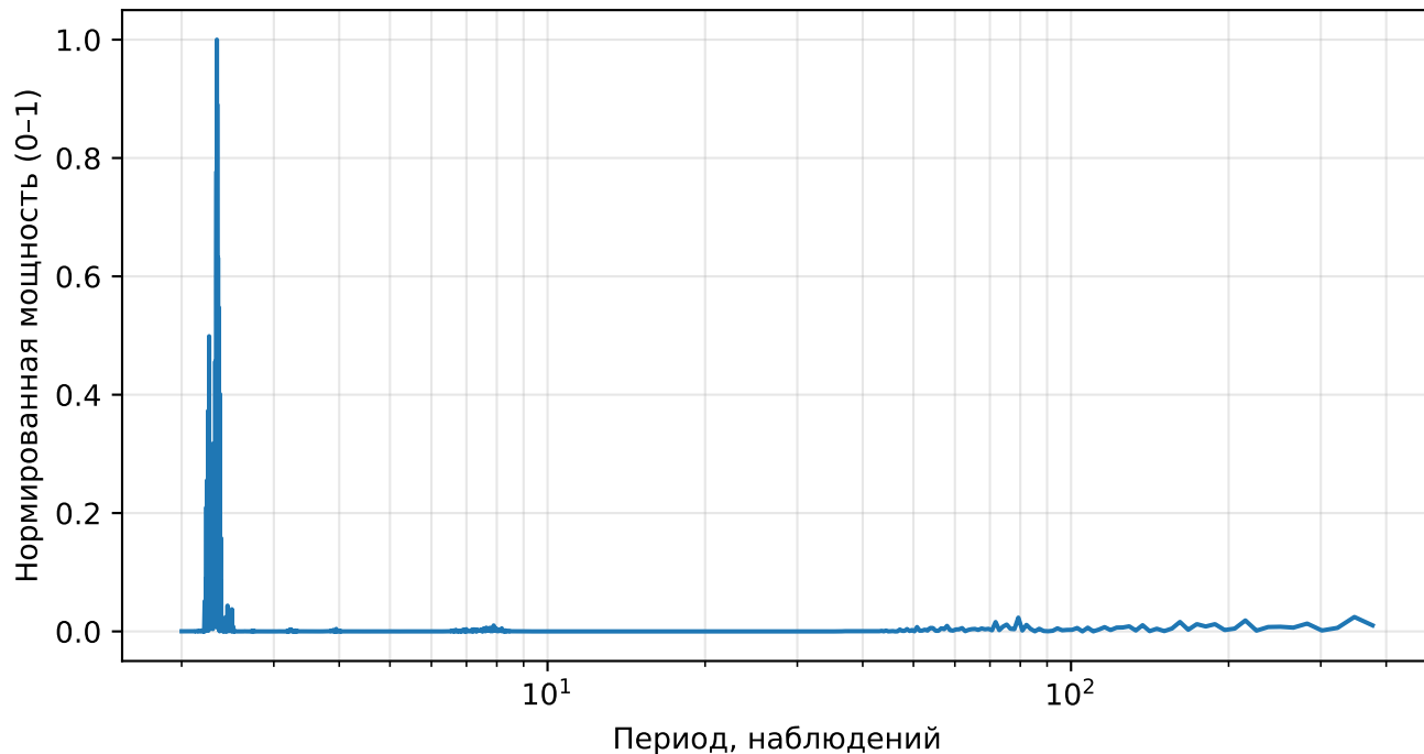
Нормированный спектр реконструкции (AE), returns, тикер: CMI
