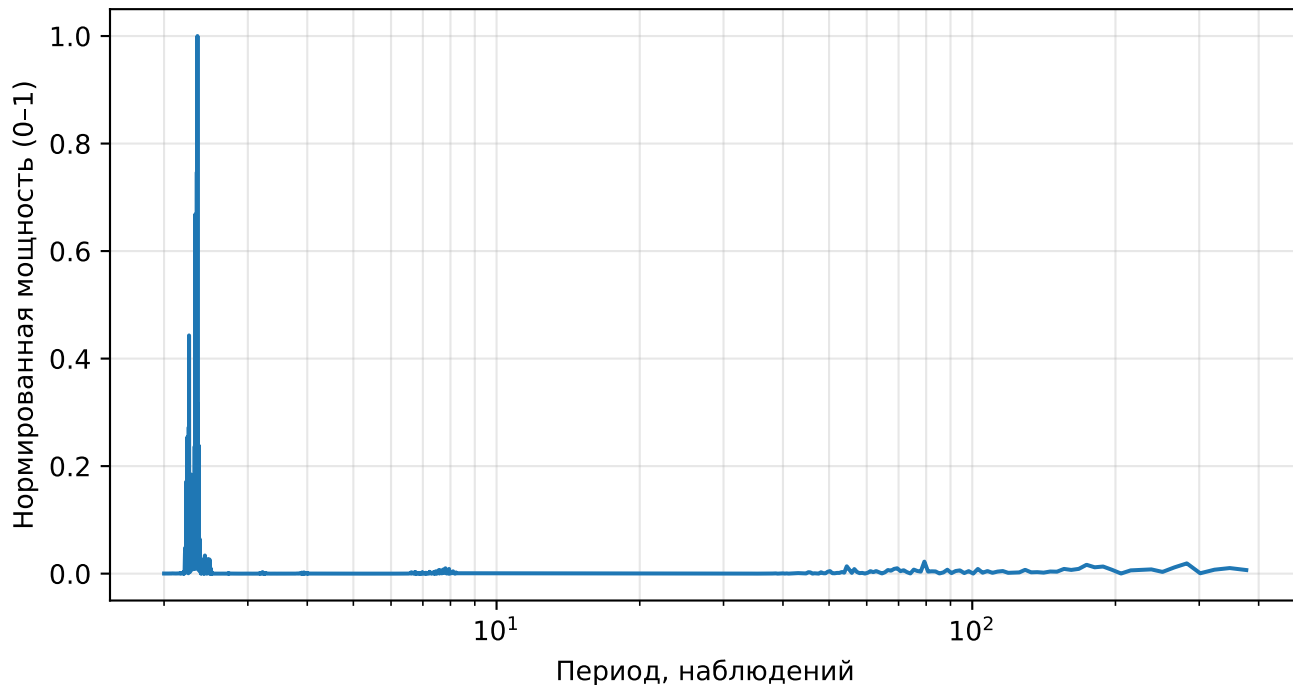
Нормированный спектр реконструкции (AE), returns, тикер: DE
