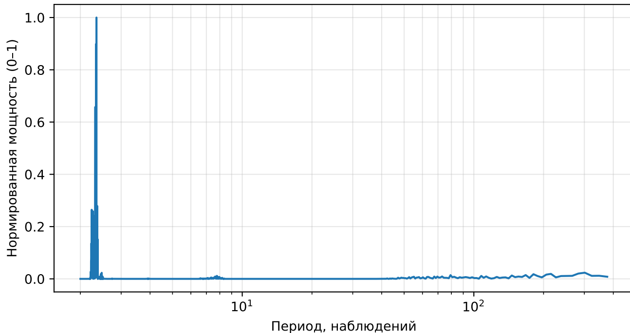
Нормированный спектр реконструкции (AE), returns, тикер: DUK
