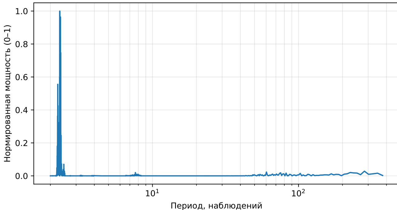
Нормированный спектр реконструкции (AE), returns, тикер: VZ
