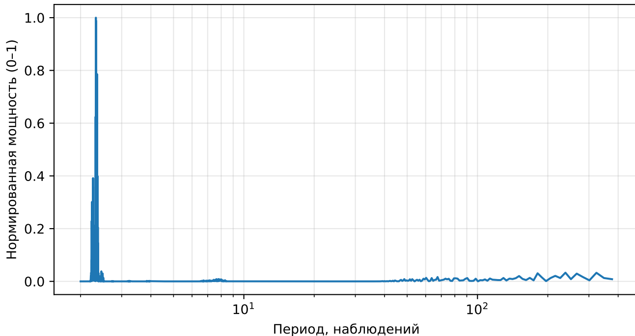
Нормированный спектр реконструкции (AE), returns, тикер: NEE
