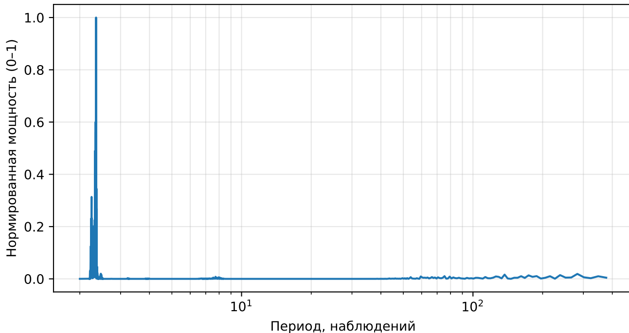
Нормированный спектр реконструкции (AE), returns, тикер: APH
