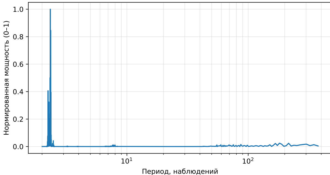
Нормированный спектр реконструкции (AE), returns, тикер: LOW
