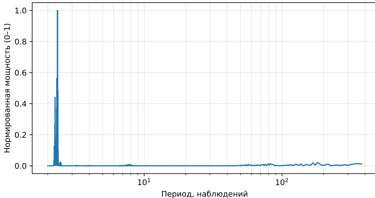
Нормированный спектр реконструкции (AE), returns, тикер: MA
