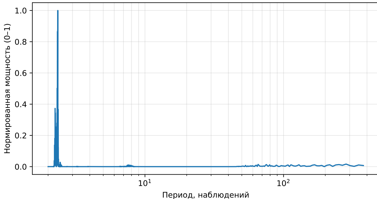
Нормированный спектр реконструкции (AE), returns, тикер: LRCX
