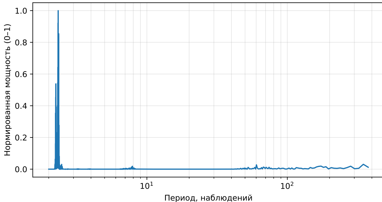
Нормированный спектр реконструкции (AE), returns, тикер: AMGN
