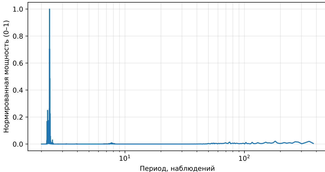
Нормированный спектр реконструкции (AE), returns, тикер: CVX
