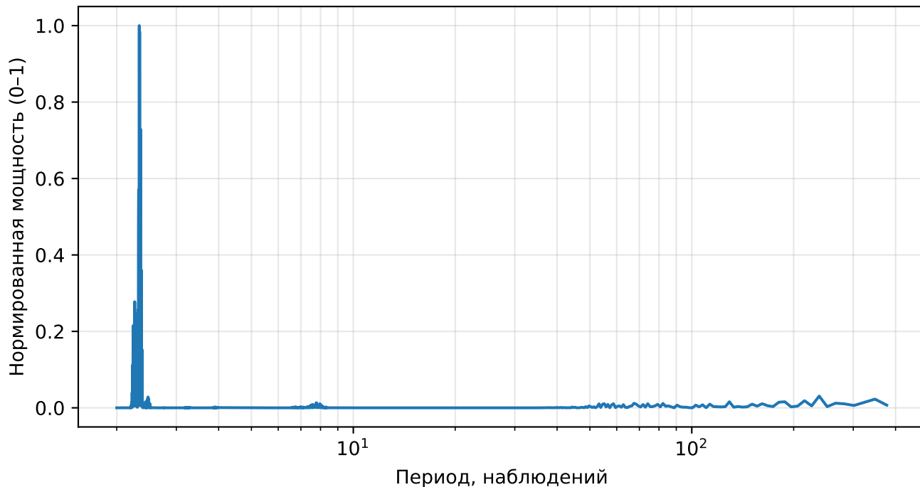
Нормированный спектр реконструкции (AE), returns, тикер: MET
