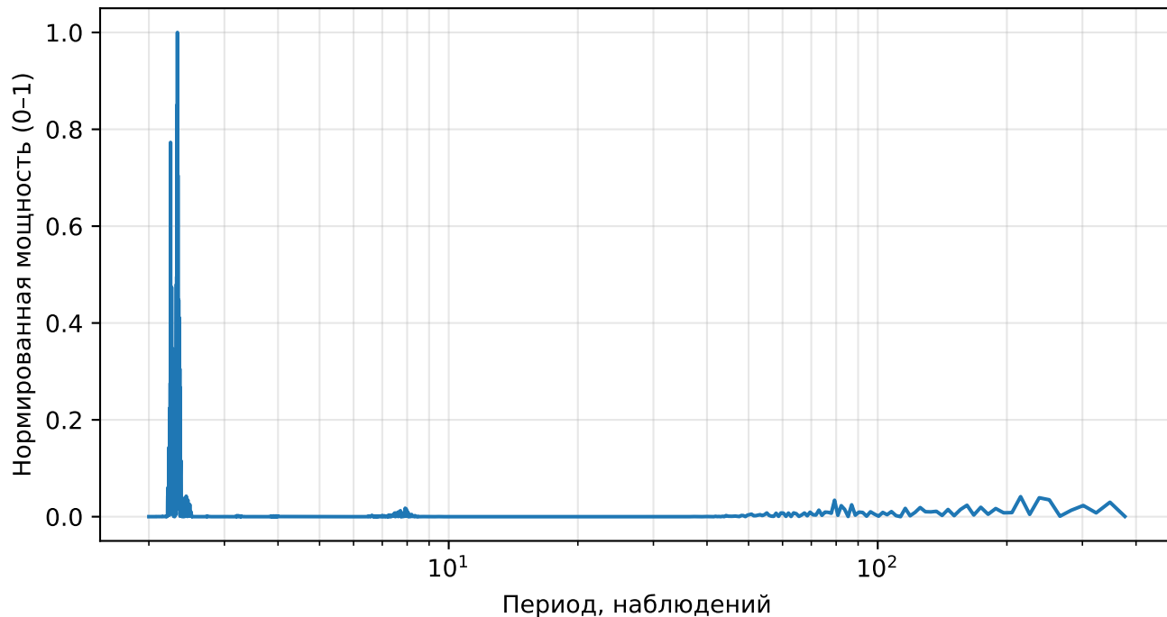
Нормированный спектр реконструкции (AE), returns, тикер: COF
