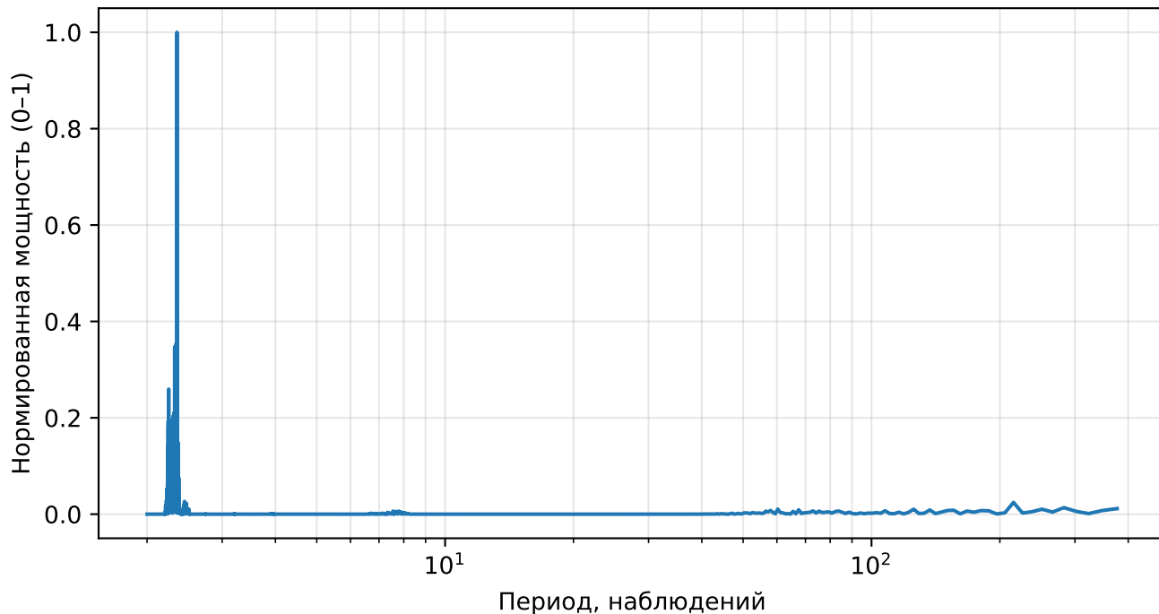
Нормированный спектр реконструкции (AE), returns, тикер: MRK
