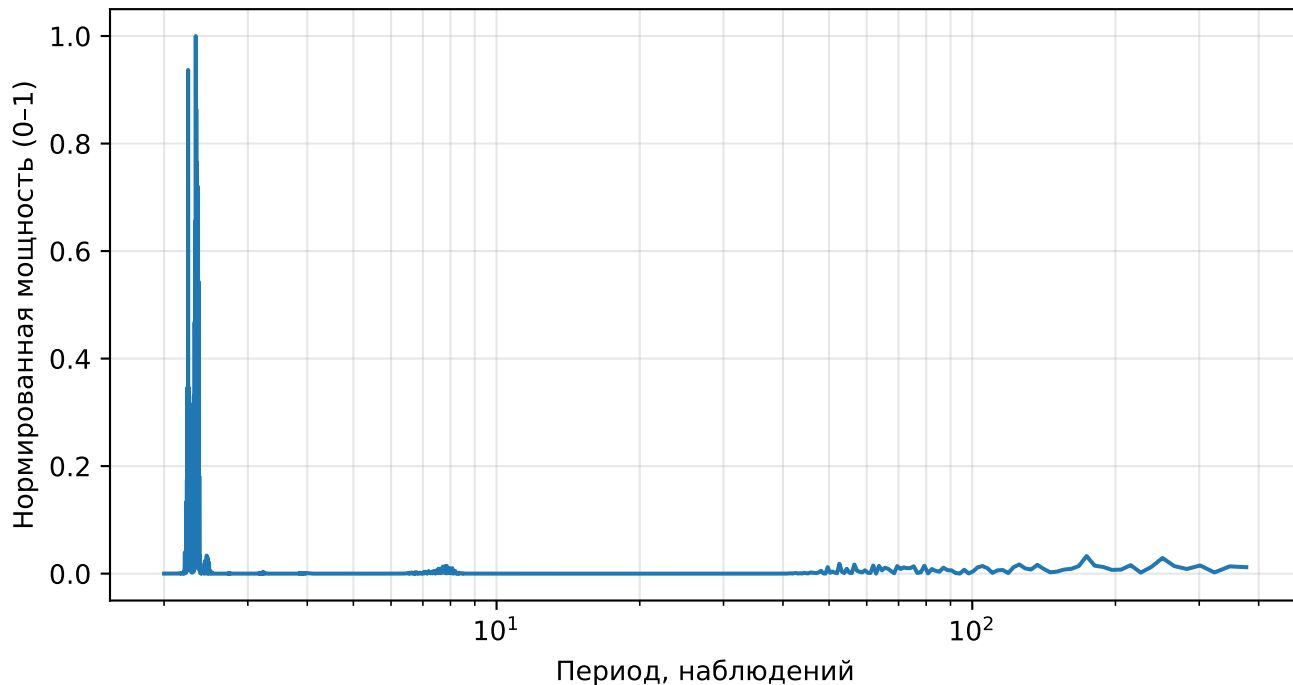
Нормированный спектр реконструкции (AE), returns, тикер: INTU
