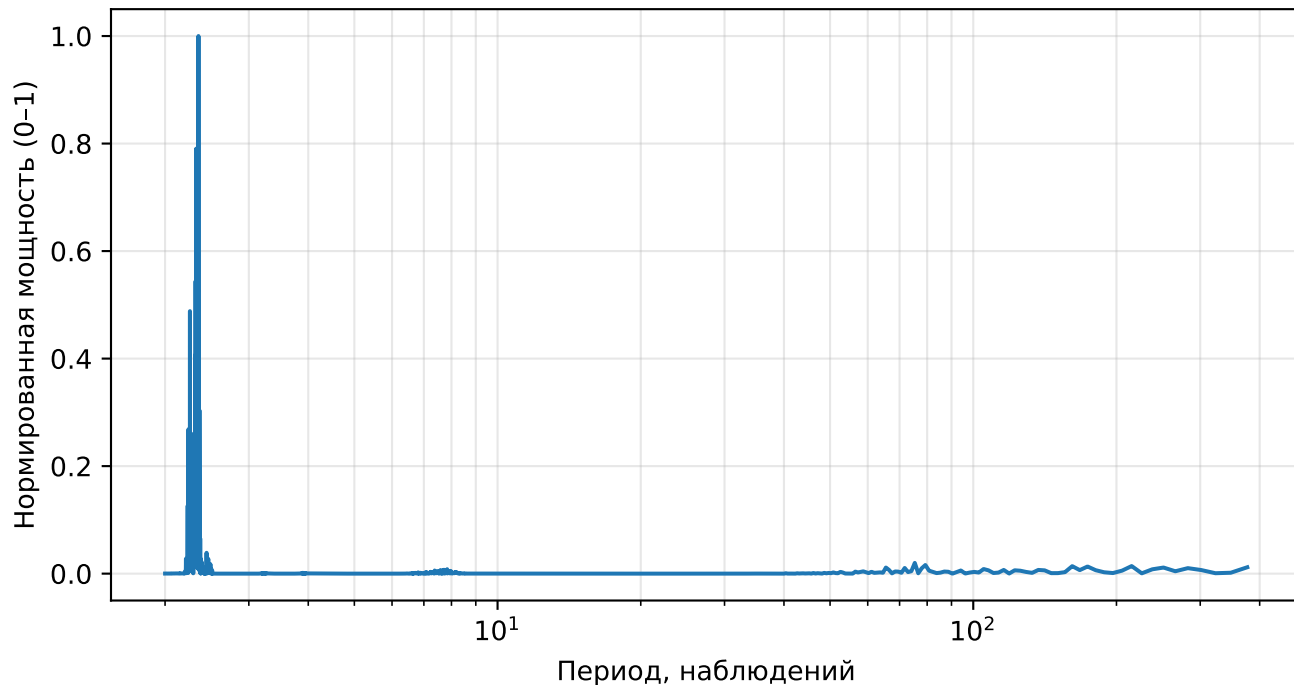
Нормированный спектр реконструкции (AE), returns, тикер: NVDA
