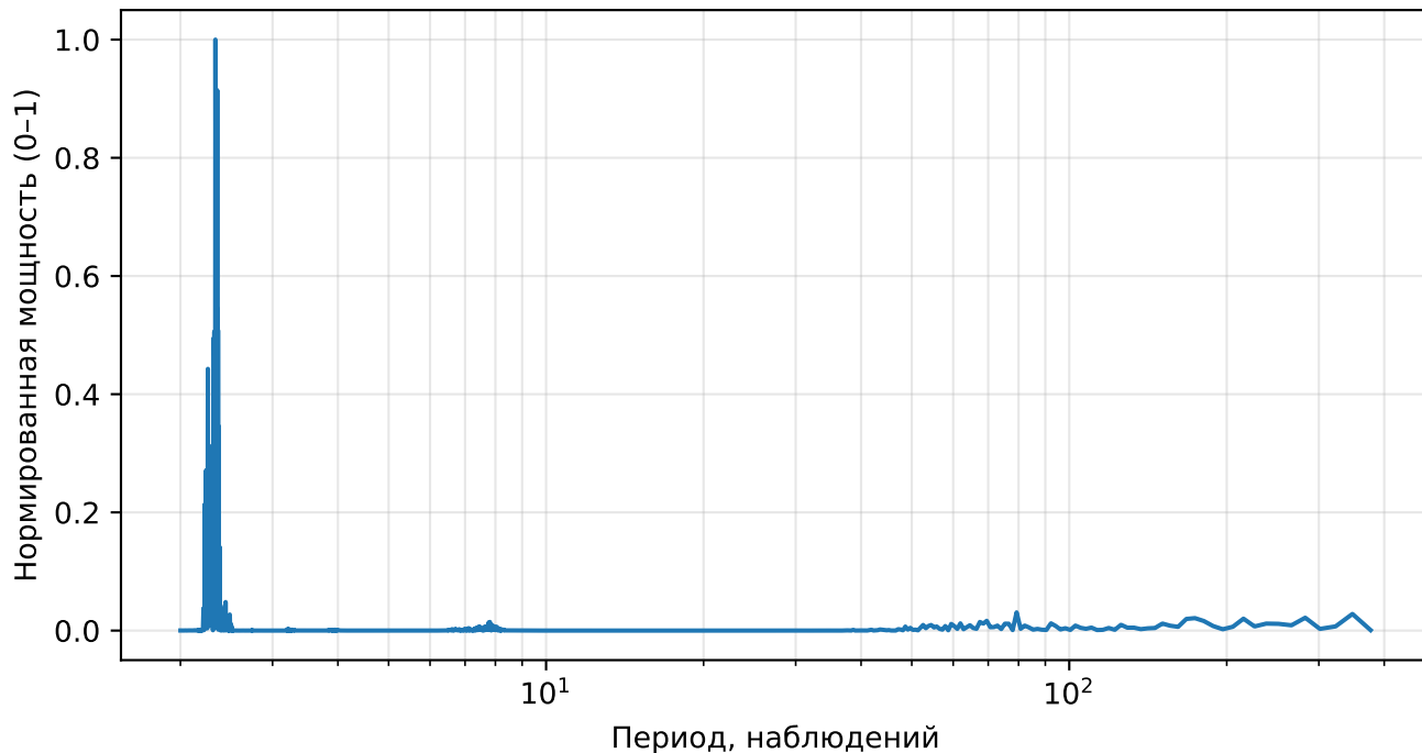
Нормированный спектр реконструкции (АЕ), returns, тикер: UNP
