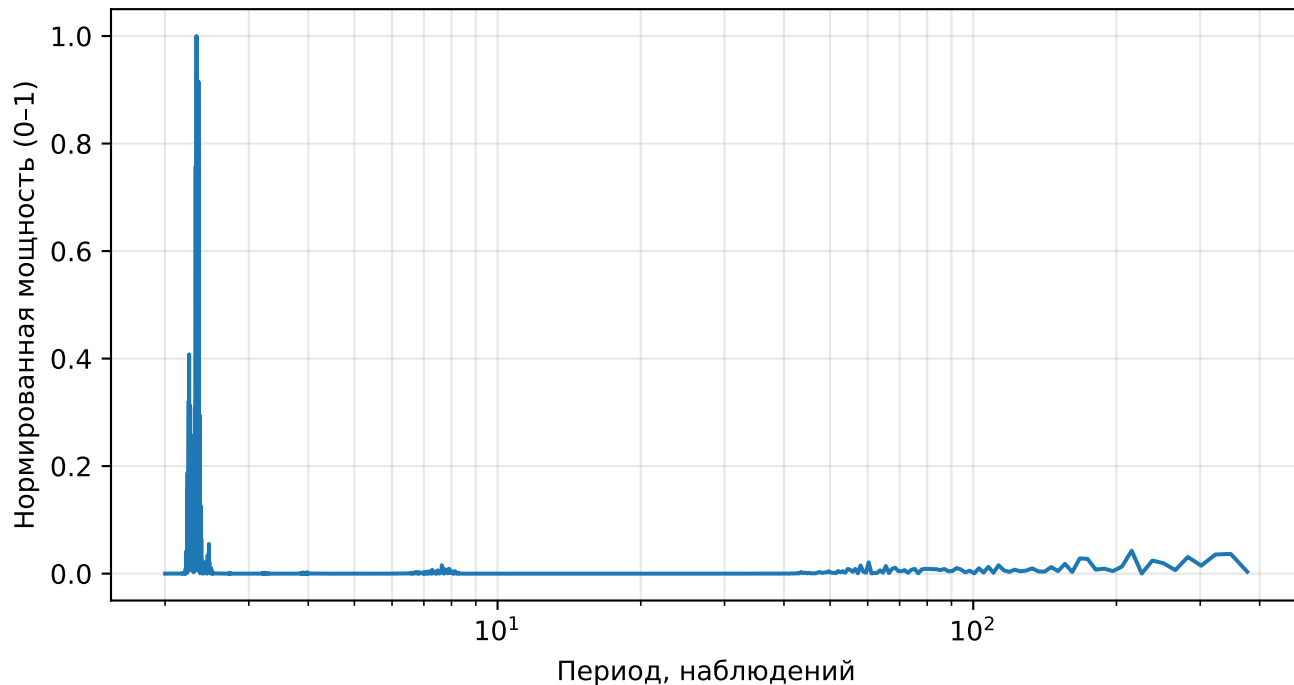
Нормированный спектр реконструкции (AE), returns, тикер: WELL
