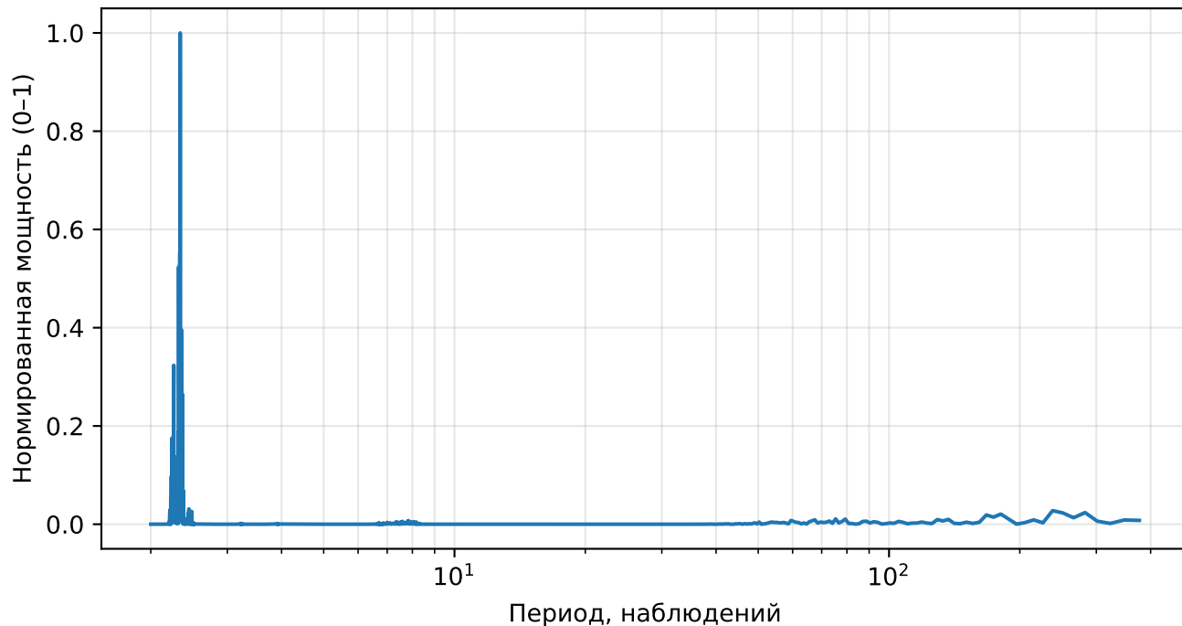
Нормированный спектр реконструкции (AE), returns, тикер: AZO
