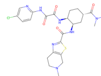
Edoxaban
