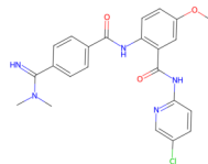
Betrixaban
