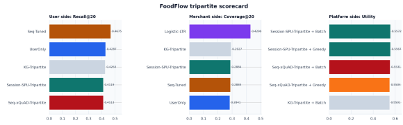
(b) 三方策略综合得分
