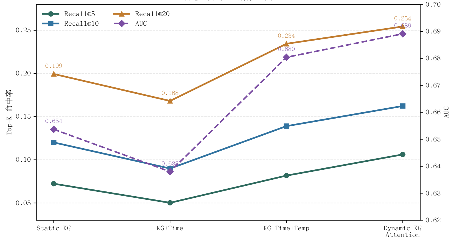
动态图谱模块消融趋势
