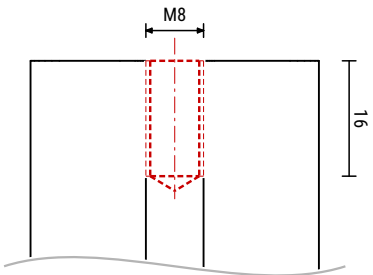
M8x16
