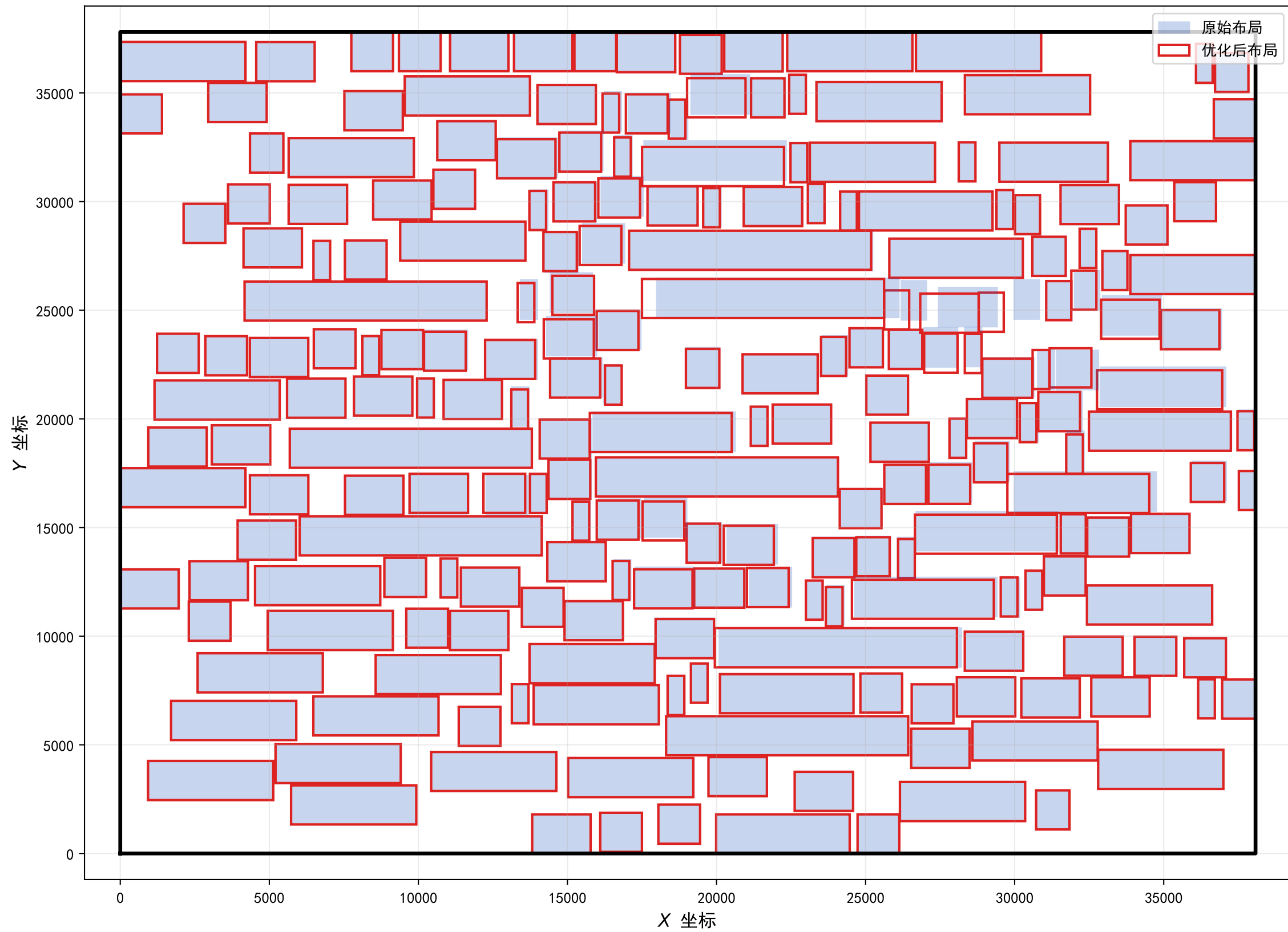
车间设备布局优化前后对比（含接口偏置与绑定）
