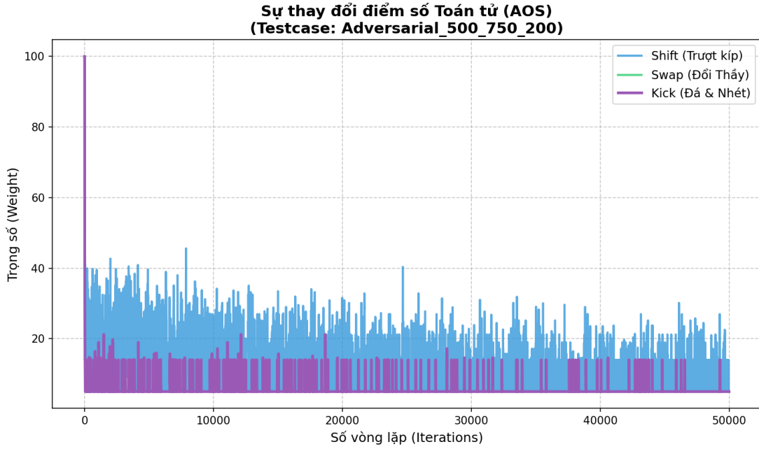
Hình 14: Sự thay đổi trọng số các toán tử Shift, Swap và Kick trong AOS-HCLS trên bộ dữ liệu Adversarial_500_750_200
