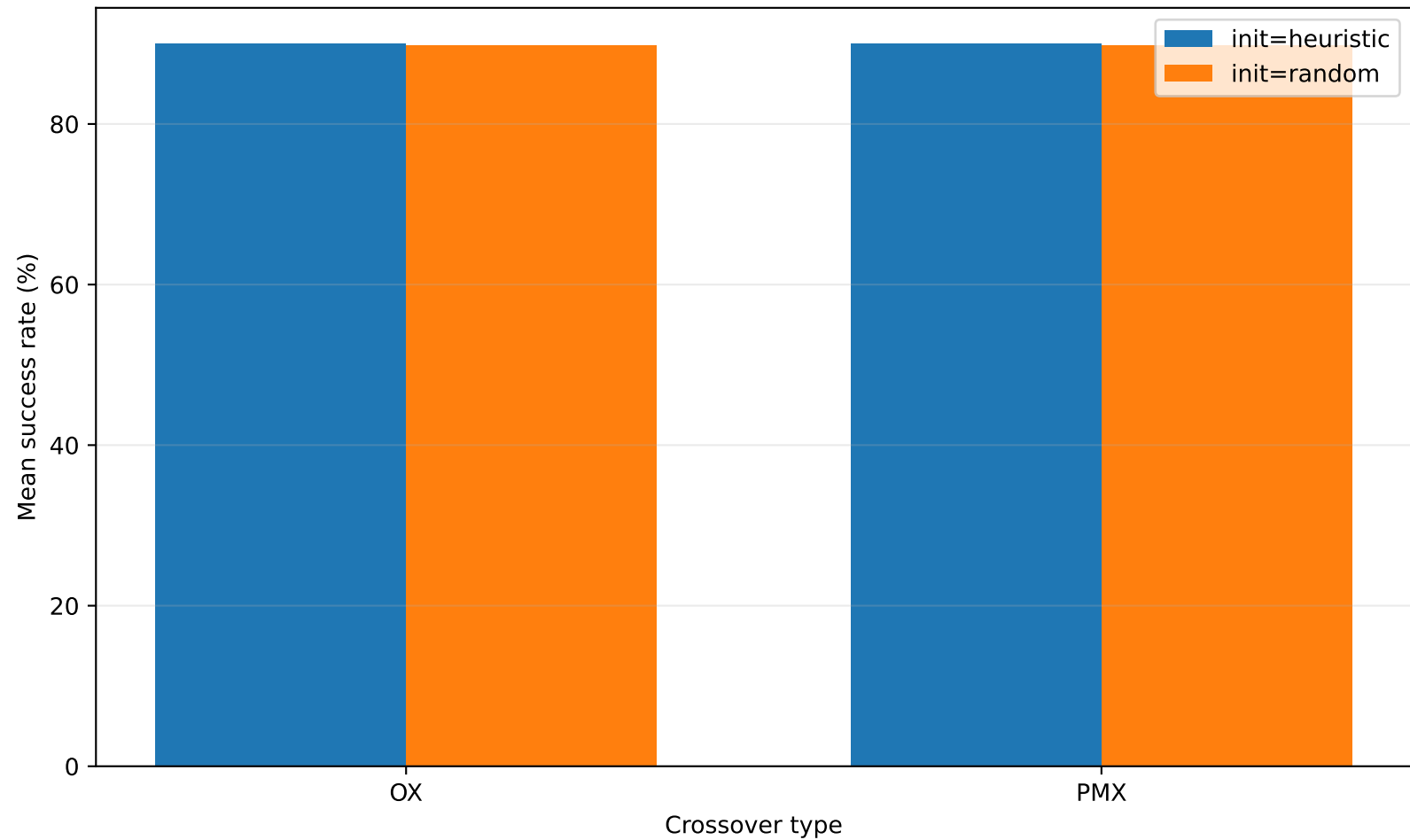
So sánh OX và PMX trên chromosome dạng hoán vị
