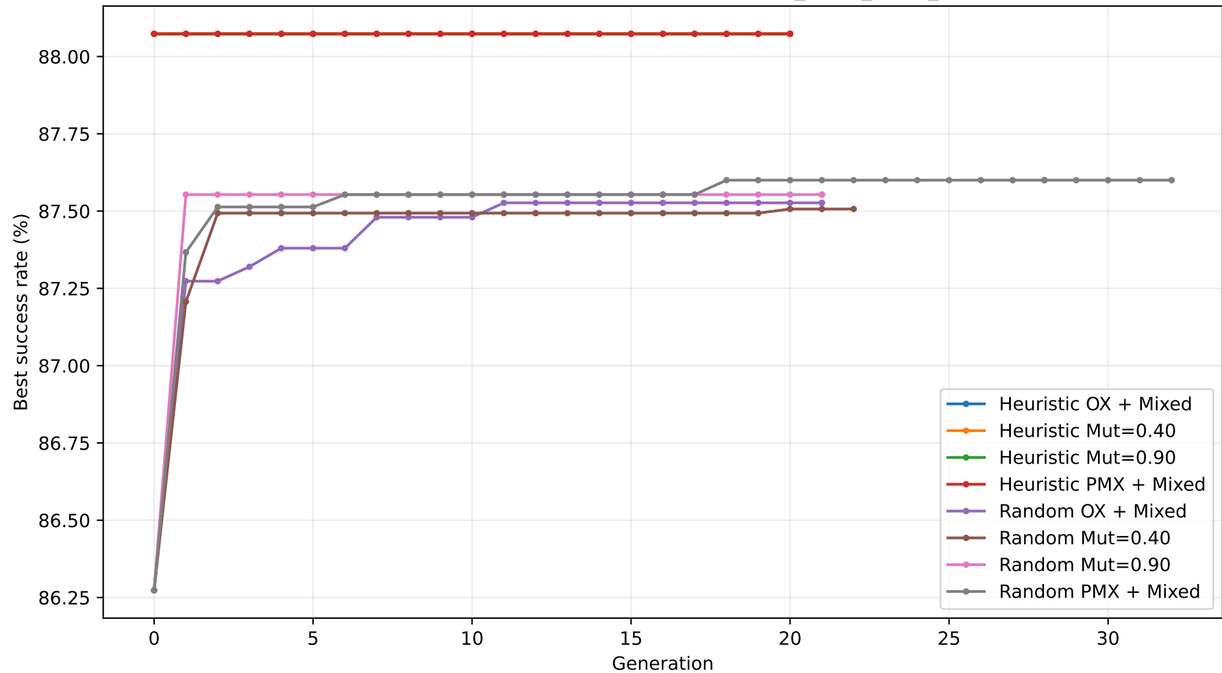
Đường hội tụ GA: Adversarial/Adversarial_1000_1500_400
