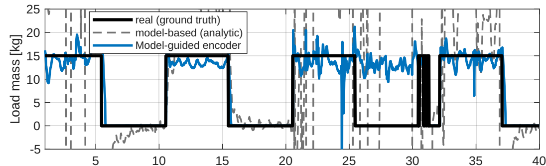
Model-guided — 负载质量/质心 估计时域 (15kg 循环负载, 滚动 vx0.5)
