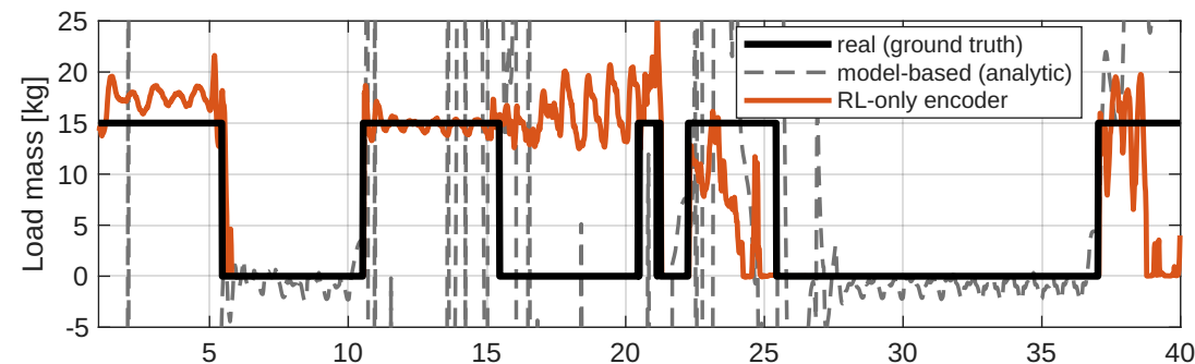
RL-only — 负载质量/质心 估计时域 (15kg 循环负载, 滚动 vx0.5)
