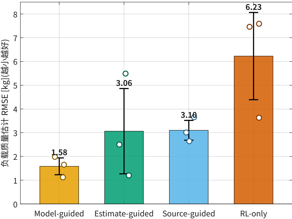
各方案负载质量估计精度(3 seed 均值 \pm 标准差,空心点=各 seed)
