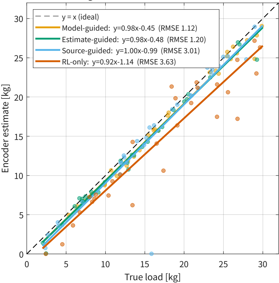
2-30 kg 负载范围内各方案的负载质量估计精度
