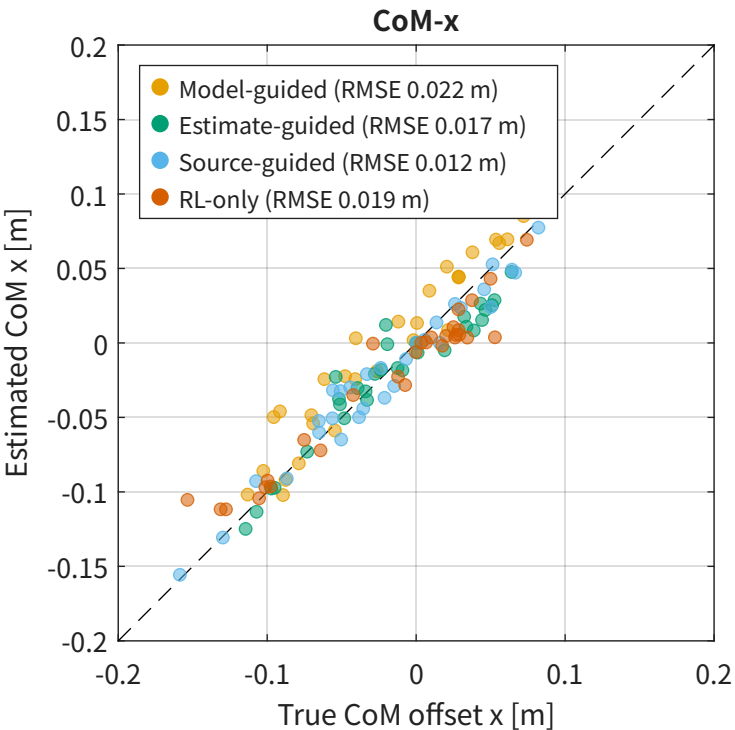
2-30 kg 负载范围内各方案对负载质心 x、y 向偏移的估计精度
