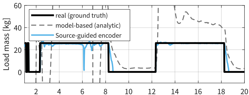
固定 26 kg 负载下 Source-guided 的负载质量与质心估计时间序列
