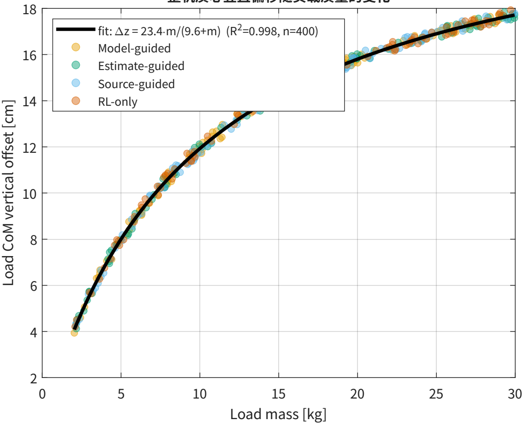
整机质心竖直偏移随负载质量的变化
