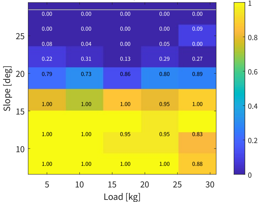
Source-guided 与 RL-only 在不同坡度与负载下的抗倾覆成功率
