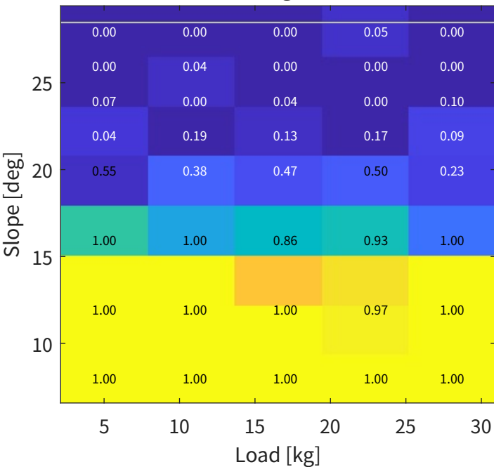
Source-guided 与 RL-only 在不同坡度与负载下的抗倾覆成功率
