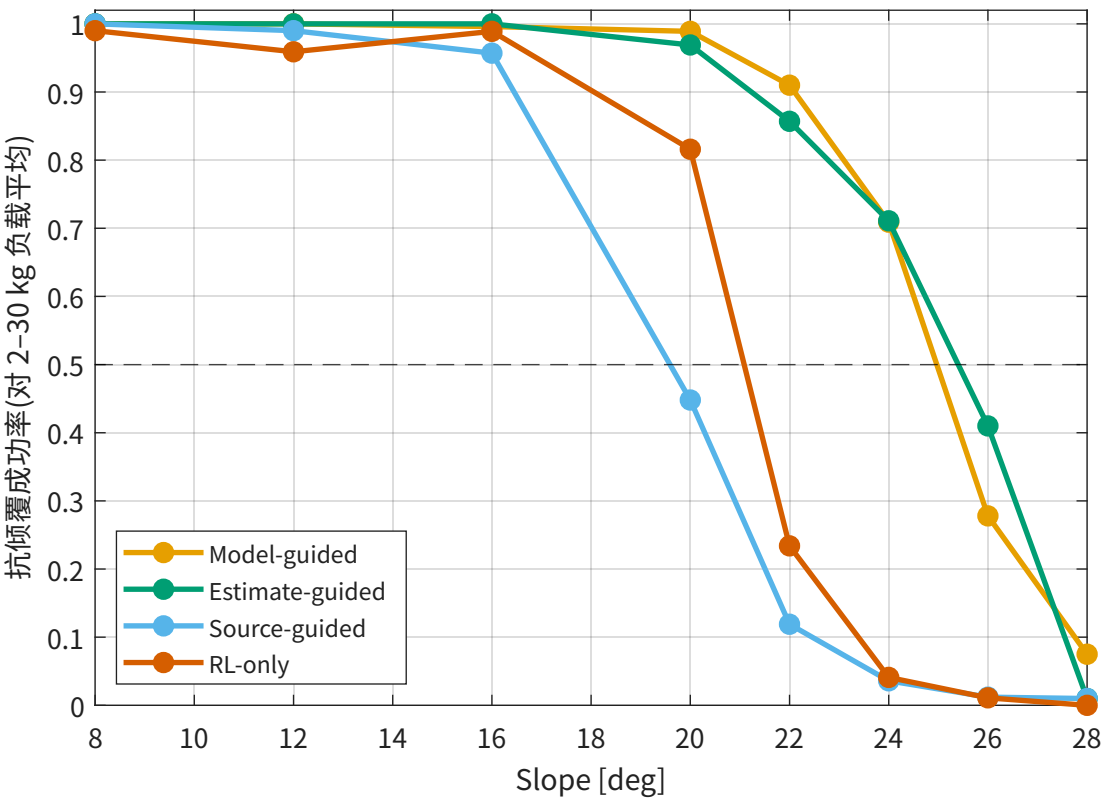
对各负载平均的抗倾覆成功率随坡度的变化
