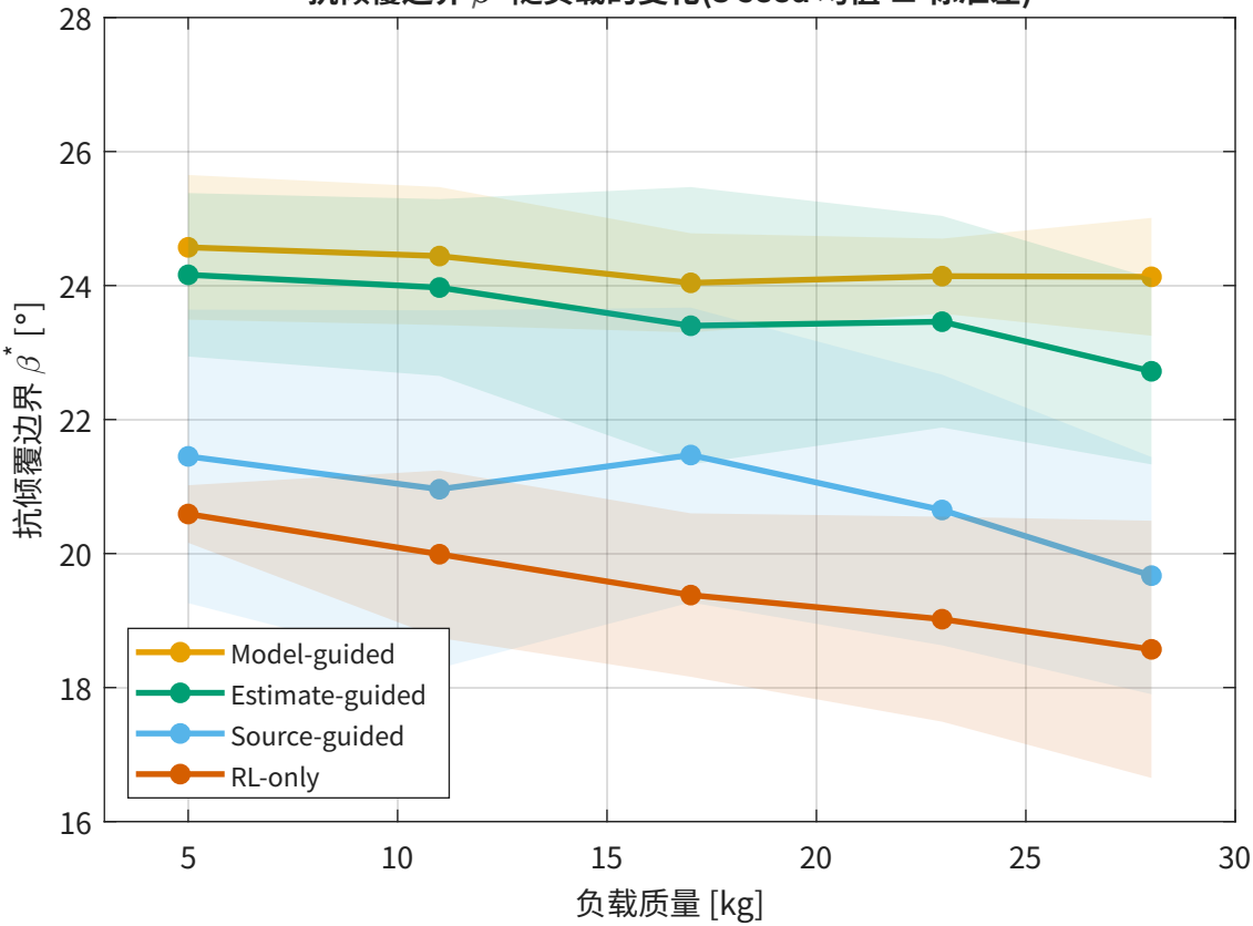
抗倾覆边界 \beta^* 随负载的变化(3 seed 均值 \pm 标准差)
