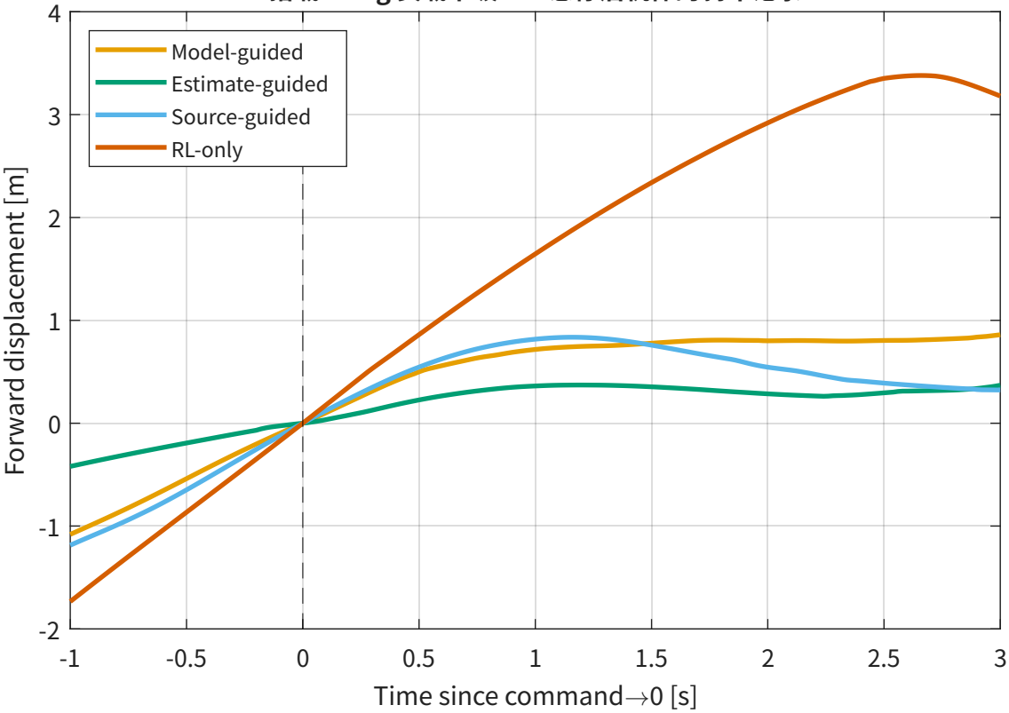
搭载 26 kg 负载下坡 10° 急停后机体的刹车记录
