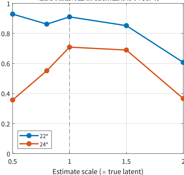
缩放负载估计量级对抗倾覆成功率的影响
