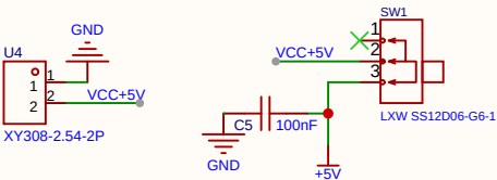
语音控制电路
