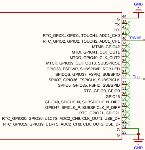
主控模块ESP32-S3-DevKitC-1
