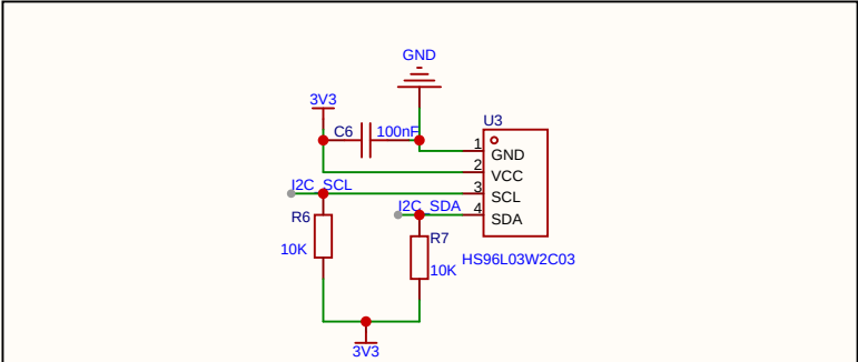
OLED显示屏
